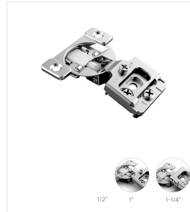
名称 美式橱柜专用缓冲铰链 快装 三维调整 Name CLIP ON 3D ADJUSTABLE AMERICAN CABINET HYDRAULIC BUFFERING HINGE
