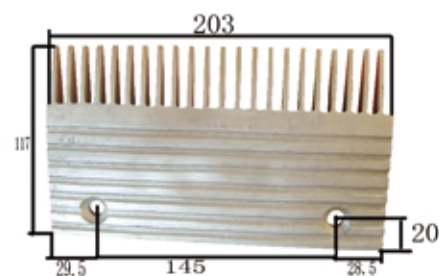
1170# 江南22齿铝梳齿板(边) 203×117×孔145 22-teeth aluminium comb plate(side)
