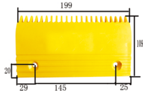
1106# 康力22齿(中) 199长 型号: BEVG KONE 22-teeth Comb (Middle)
