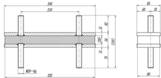
430# (SLBJ-177/B) 上梁缓冲垫 Upper beam cushion
