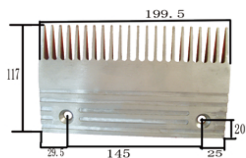
1169# 江南 22齿铝梳齿板 (中) 199.5×117×孔145 22-teeth aluminium comb plate(centre)
