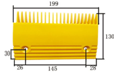
1111# 东芝22齿ABS梳齿板 (中) 199×130×孔145 22-teeth ABS comb plate (left, centre)
