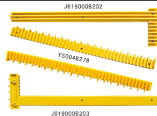
959# 三菱扶梯边框二代 Mitsubishi Escalator Frame II
