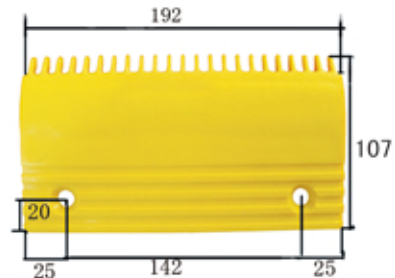
1097# 西子OTIS 23齿塑料梳齿板 (中) 192×107×孔142 识别号(Number of Identification) LDTJ-B-3 23-teeth plastic comb plate(centre)
