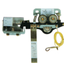
332# 广日门锁 Guang Ri door lock
