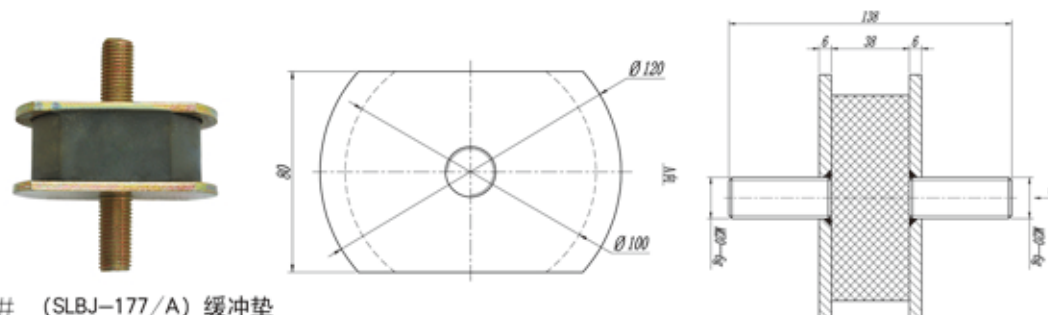
429# (SLBJ-177/A) 缓冲垫 crash pad
