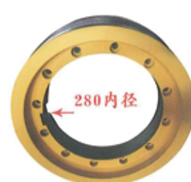
693# 西子富沃德曳引轮 400×5×10/400×6×10 Xizi fouwald traction wheel
