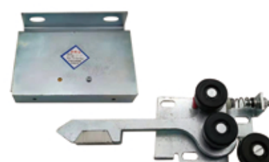
210# 奥的斯09门锁 Otis 09, door lock
