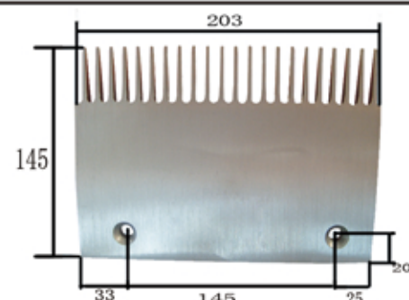
1186# 西子OTIS 22齿铝梳齿板 (左) 203×145×孔145 22-teeth aluminium comb plate(left)
