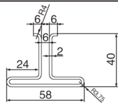
654# 实心轨T50 Solid Rail T50
