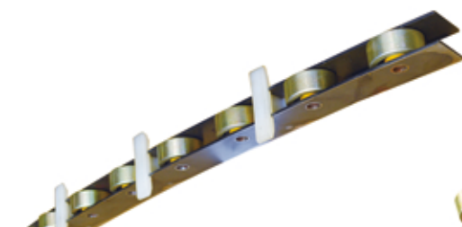
821# 长条形8轮滑轮群 全长610 轮φ41×厚17 总厚25 Pulley Group (8 Rollers) L610×T25
