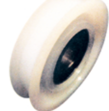
193# OTIS尼龙门 吊轮 φ85×20×6204 Otis Nylon door
