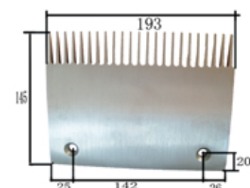
1184# 西子OTIS 23齿人行道铝梳齿板 193×145×孔142 (中) 识别号(Number of Identification) XAA453J 23-teeth aluminium comb plate(centre)
