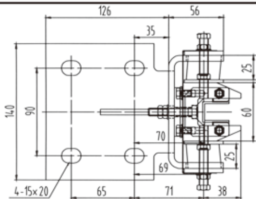
037# 固定导靴 200×16.5/10.5 Fixed Guide shoe
