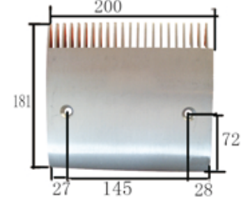
1167# 迅达9500人行道22齿铝梳齿板 200×181×孔距145 (中) 22-teeth aluminium comb plate(centre)
