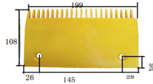
1114# 迅达22齿塑料梳齿板 (中) 199×108×孔145 22-teeth plastic comb plate (centre ,right)
