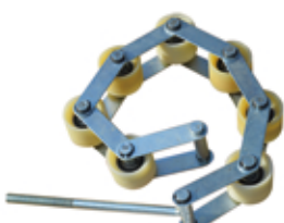
826# 百斯特涨紧总成节距 110×M18 轮φ70×50×204 M18螺丝
