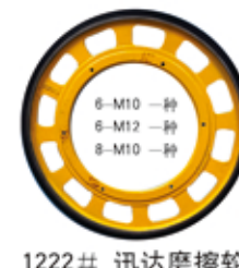
1222# 迅达摩擦轮 φ 588×内 φ 400×厚30 Schindler Friction Pulley φ 588×inner φ 400×H30
