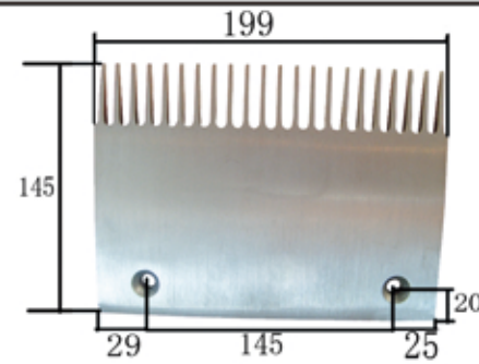
1188# 西子OTIS 22齿铝梳齿板 (中) 199×145×孔145 22-teeth aluminium com plate (centre)
