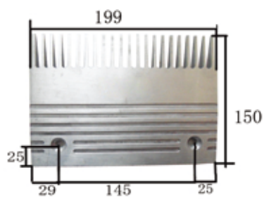
1172# 江南22齿铝梳齿板(中) 199×150×孔145 22-teeth aluminium comb plate(centre)
