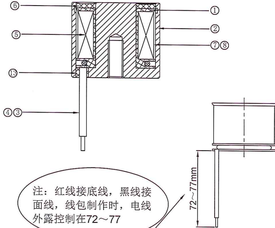
产品结构图:
