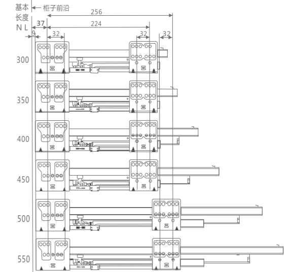
安装孔尺寸(mm)
