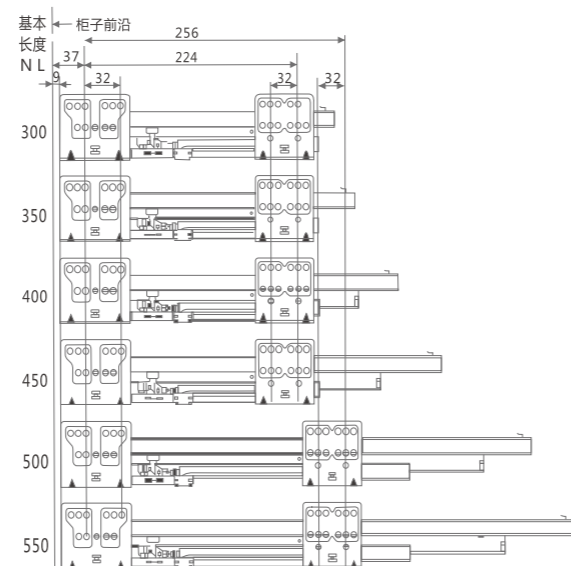
安装孔尺寸(mm)
