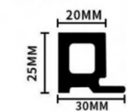
收边条
