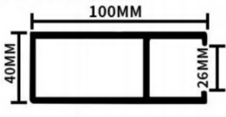
100X40天花
