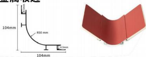
金属收边
