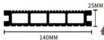
140X25方孔地板
