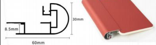
金属收边
