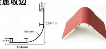
金属收边
