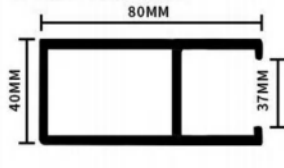
80X40天花
