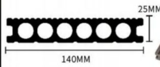
140X25圆孔地板
