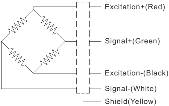
Wiring Code
