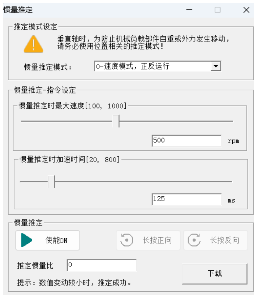
图3-42 惯量辨识
