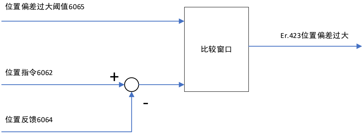
图3-57 CSP 位置偏差过大概览图
