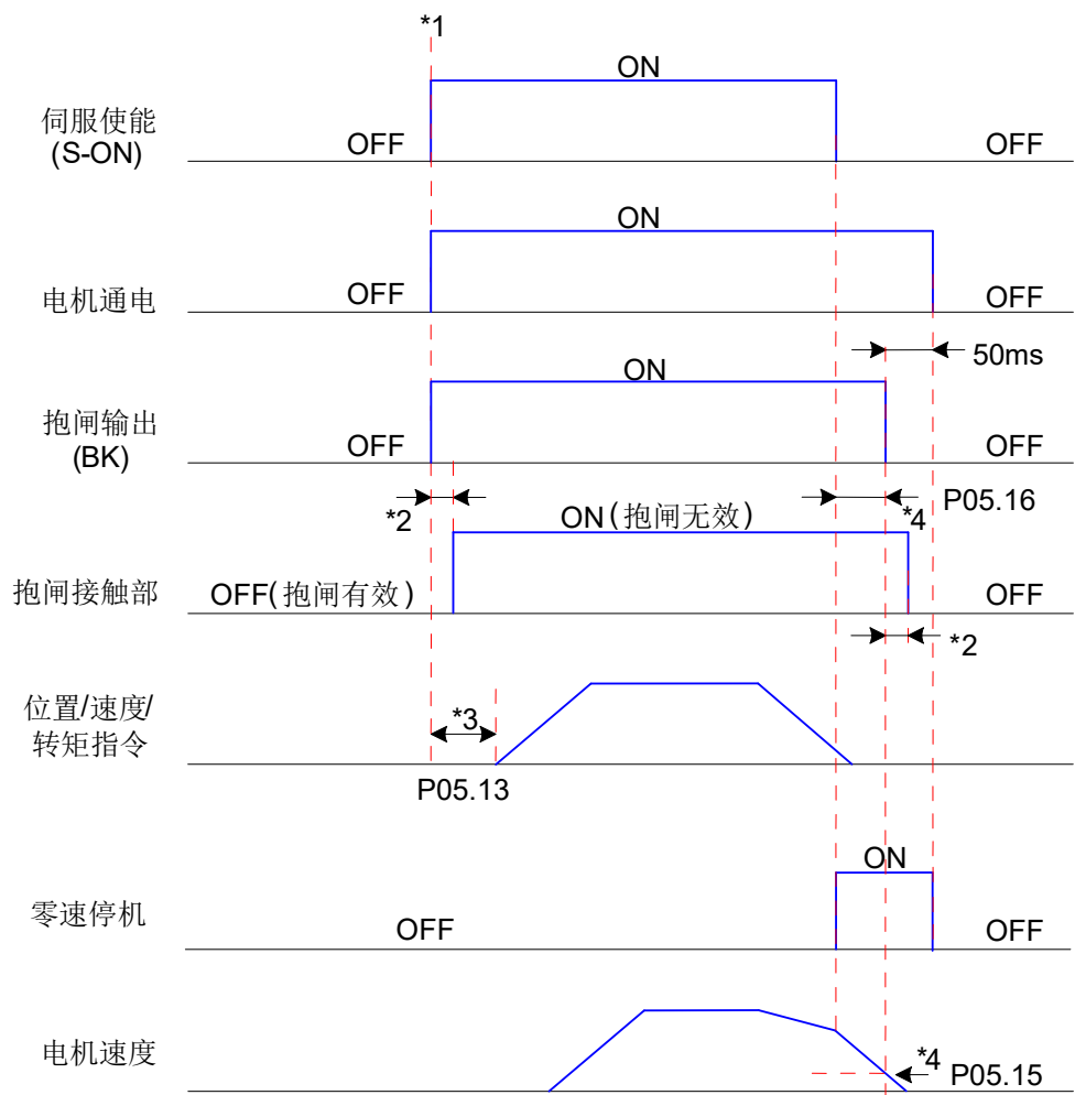
图3-4 电机运动时抱闸时序图
