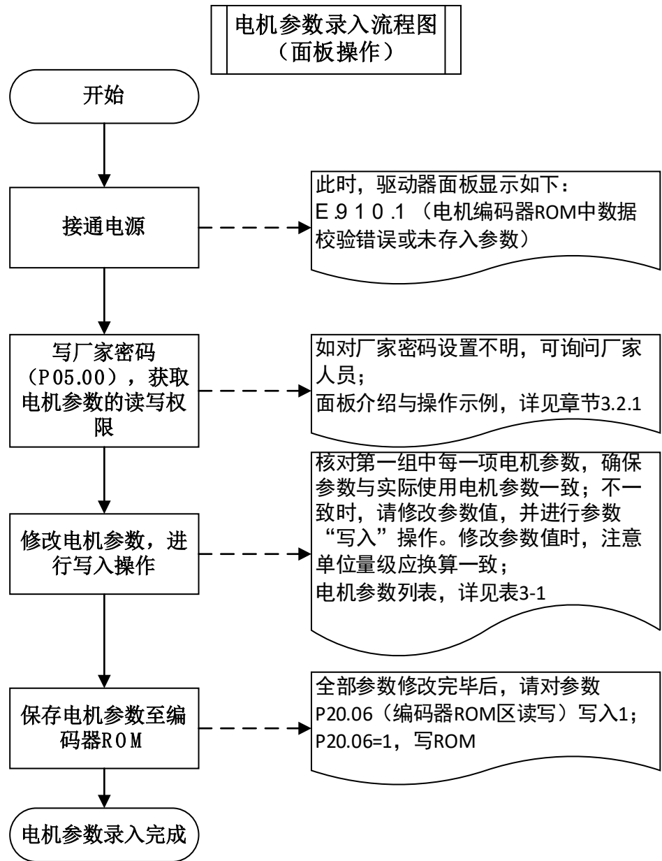
图3-1 电机参数录入面板操作流程
