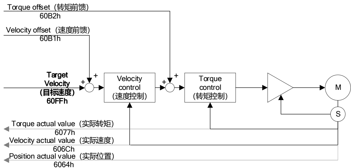
图3-59 同步周期速度模式 (CSV) 概览图
