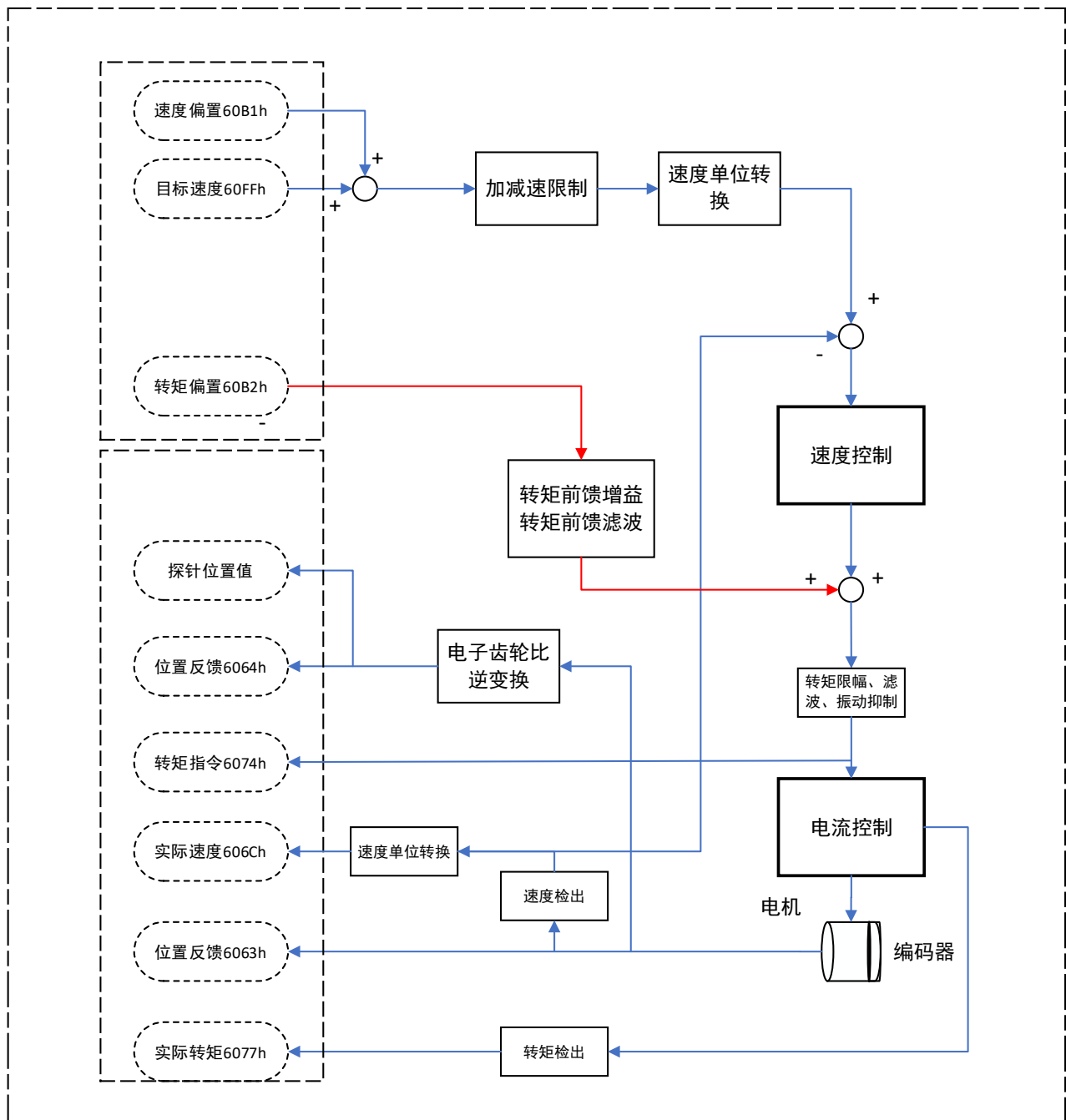
图3-60 同步周期速度模式 (CSV) 框图
