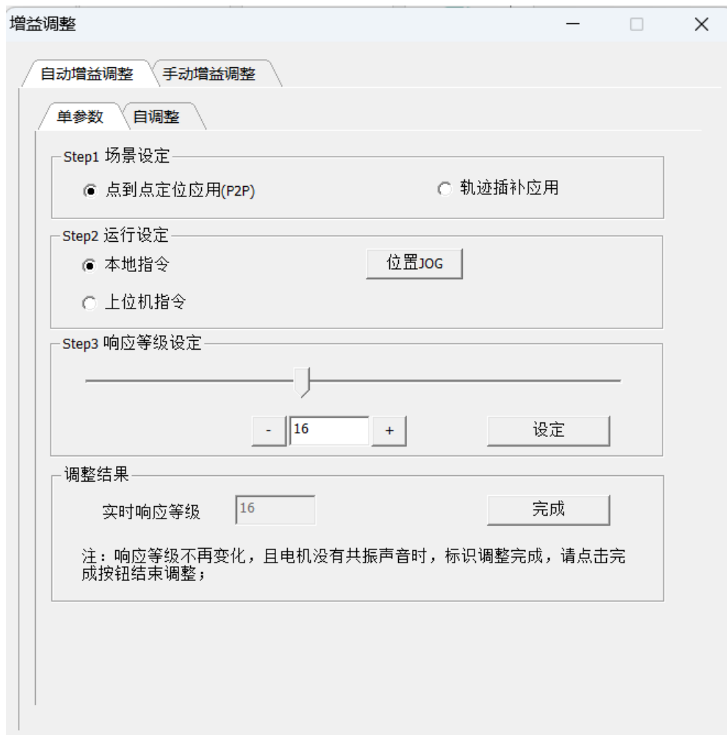
图3-43 刚性表设置
