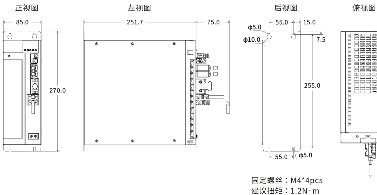
图1-8 SIZE-D 外形尺寸图 (单位 mm)
