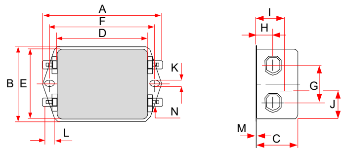
图2-30 FN 2090 系列 1-20A 滤波器尺寸图(单位: mm)
