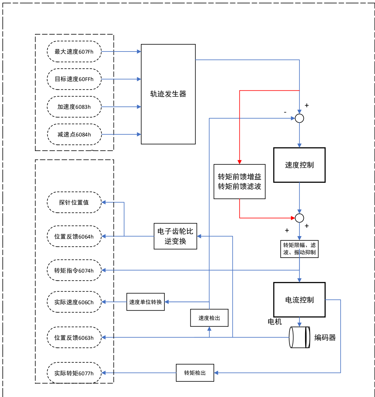
图3-69 轮廓速度模式(PV)控制框图
