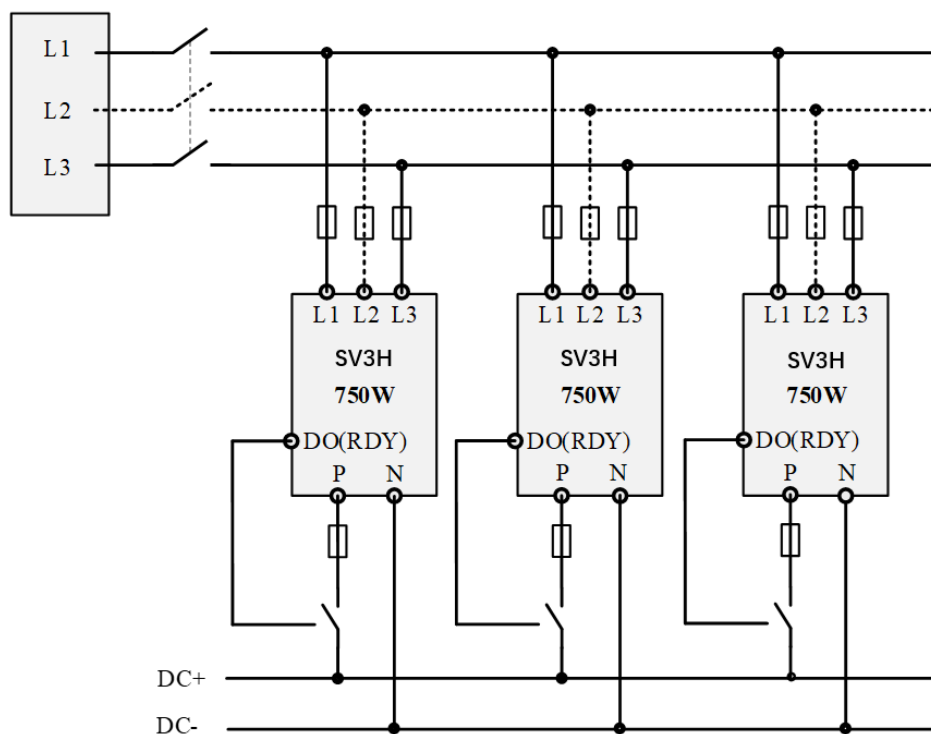
图2-10 伺服共母线示例
