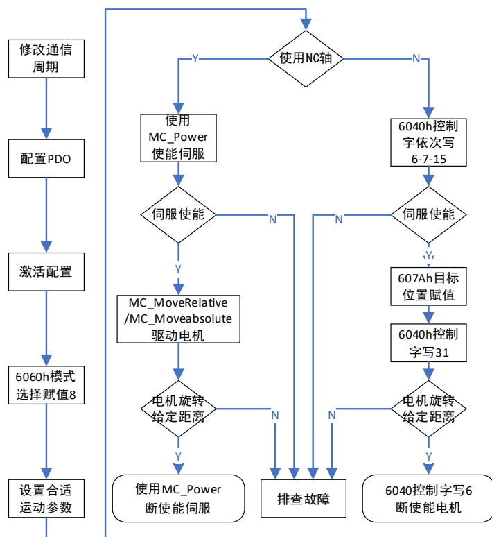
图7-21 CSP 模式使用示例流程图
