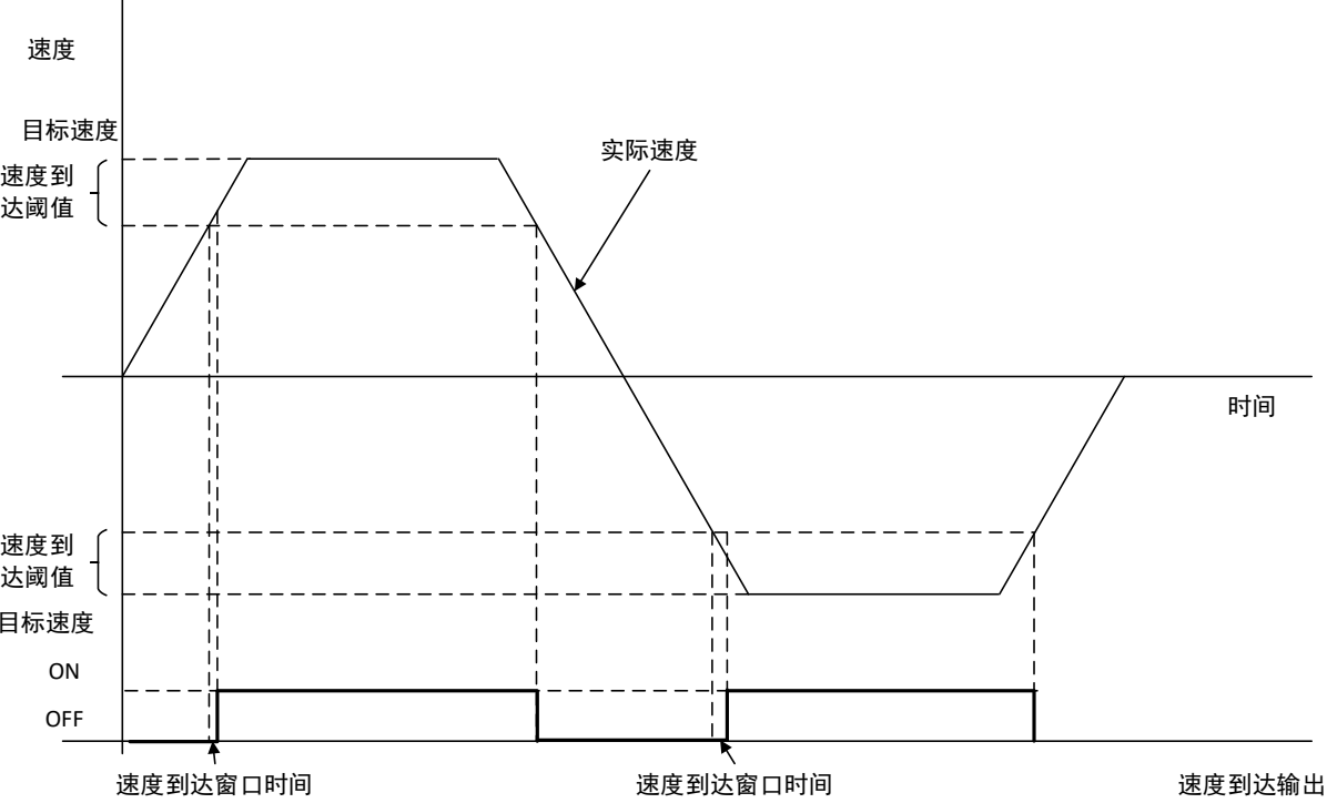
图3-61 CSV 速度到达功能示意图
