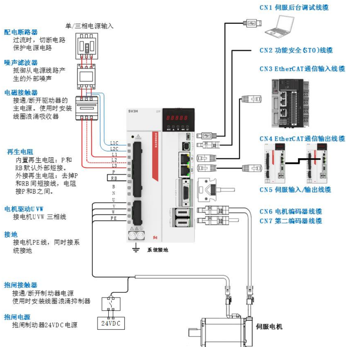
图2-3 SIZE-C 系统配线图
