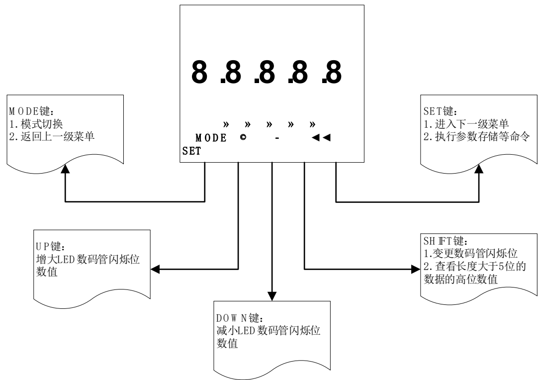
图3-15 按键功能介绍图
