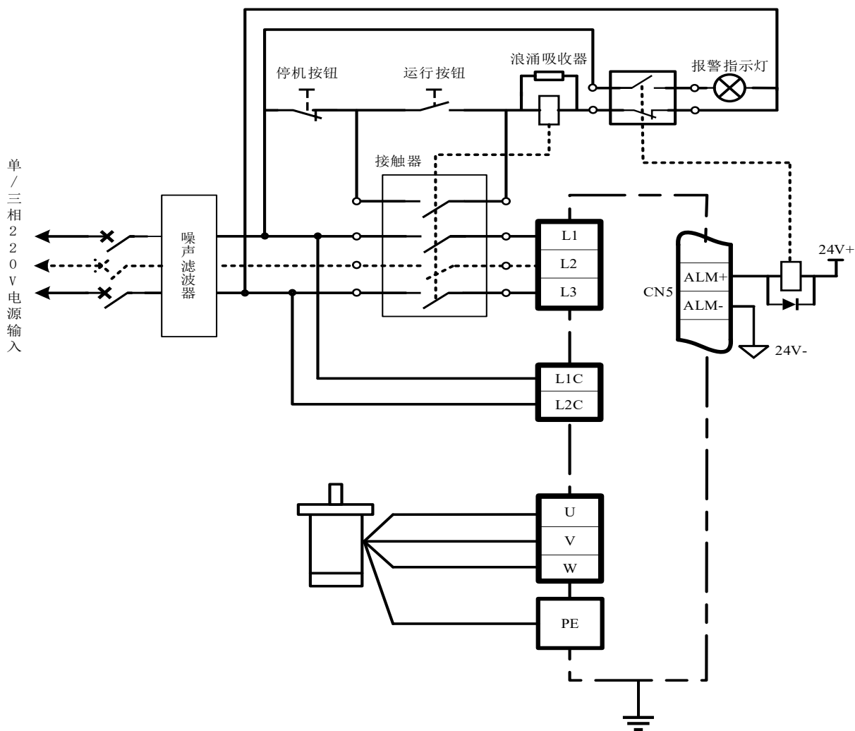
图2-7 SIZE-B 主电路配线示例
