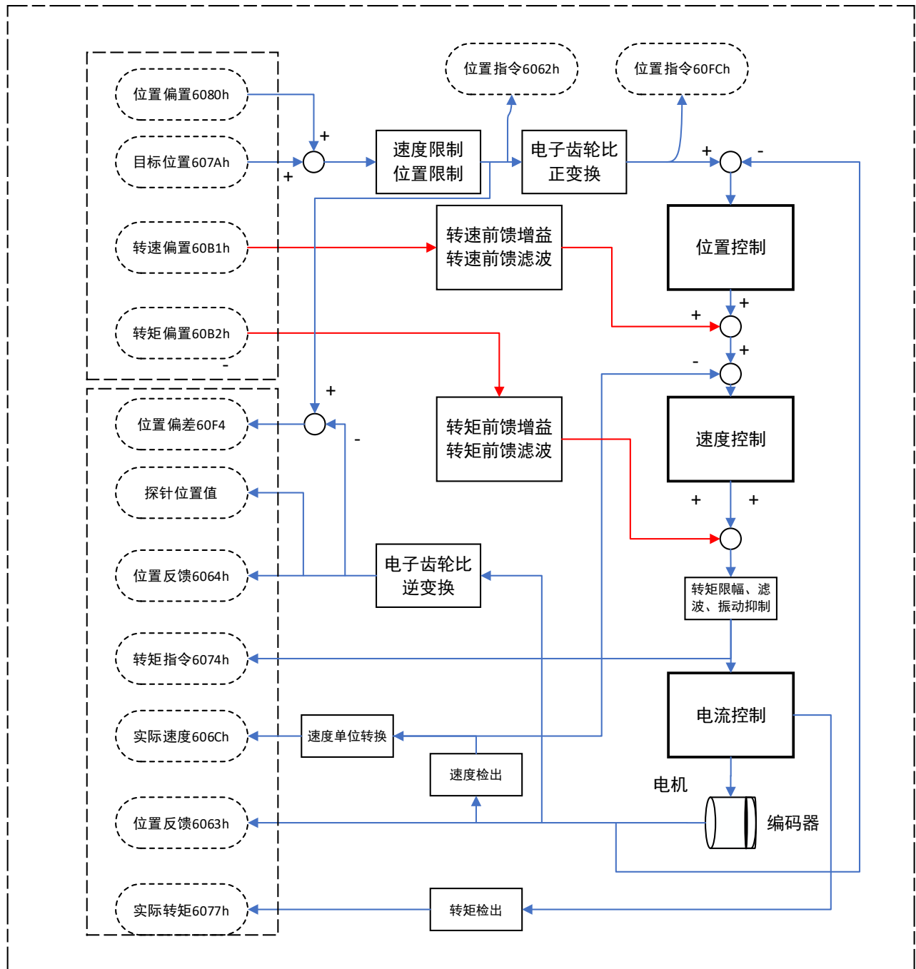
图3-54 同步周期位置模式框图
