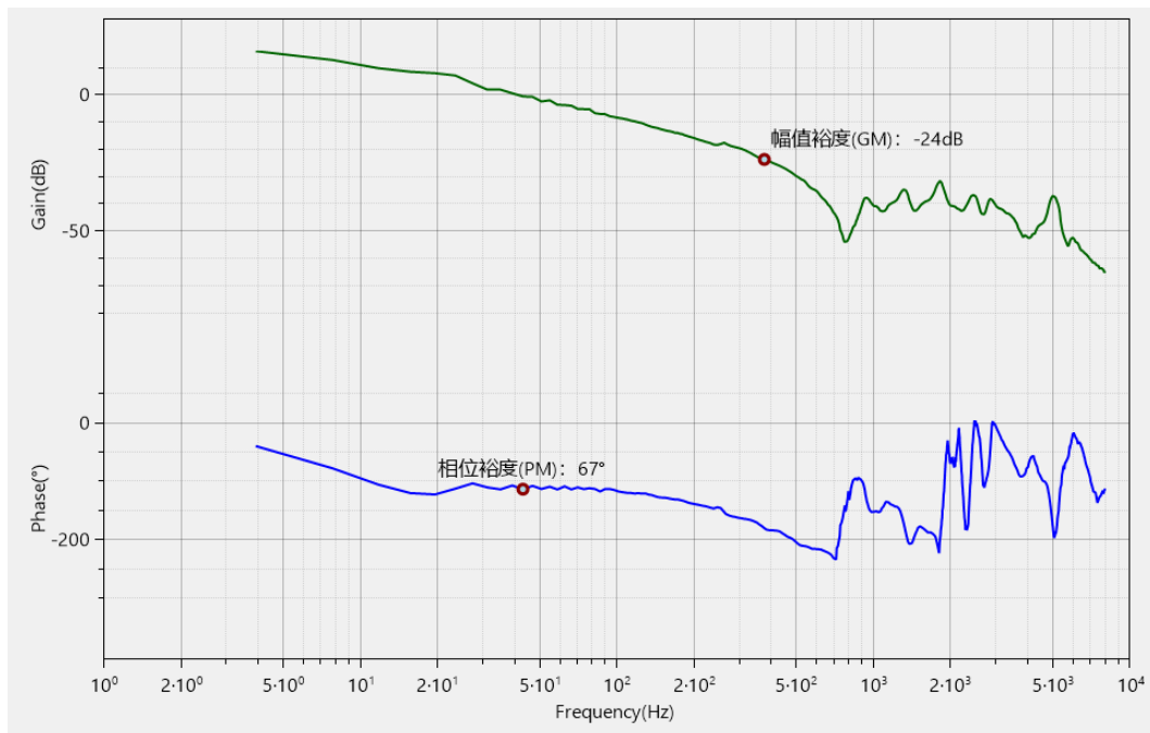
图3-46 速度开环
