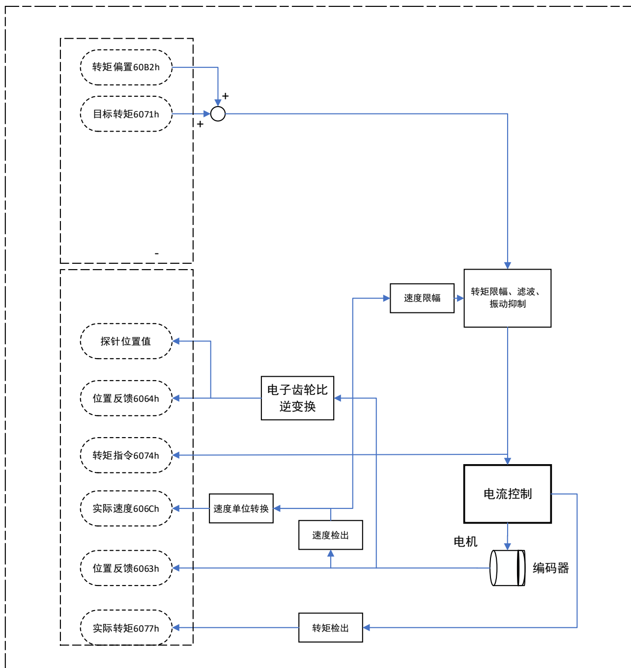
图3-63 同步周期转矩模式 (CST) 框图
