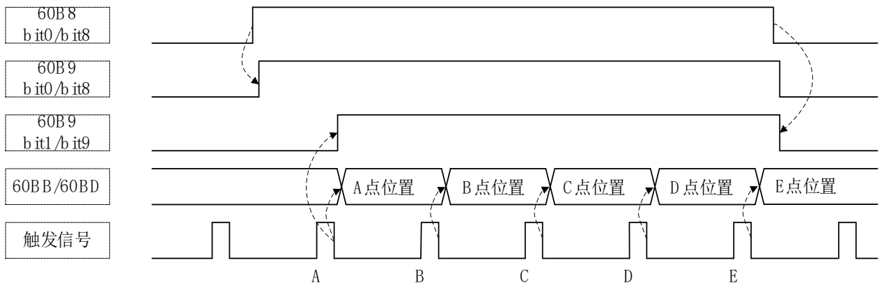
图3-79 连续下降沿锁存
