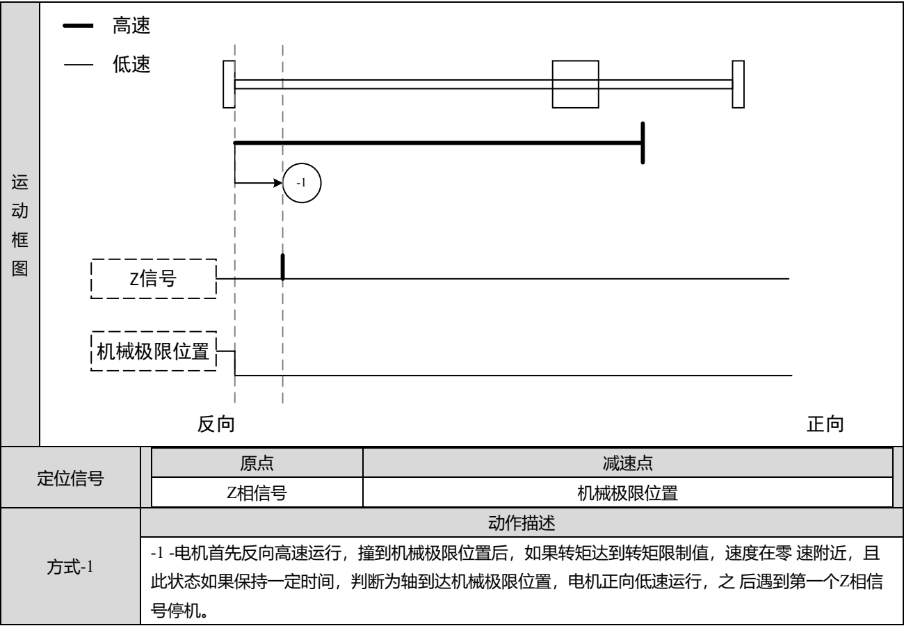
图3-74 原点复归模式 -1
