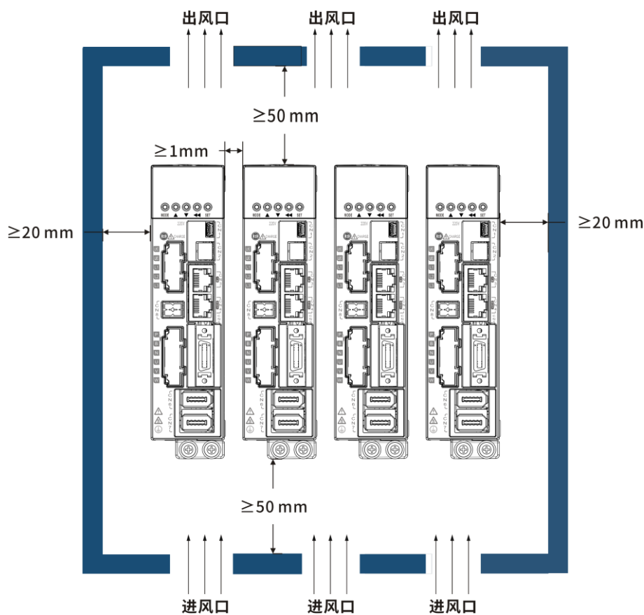
图1-10 伺服驱动器安装示意图（紧凑安装时）
