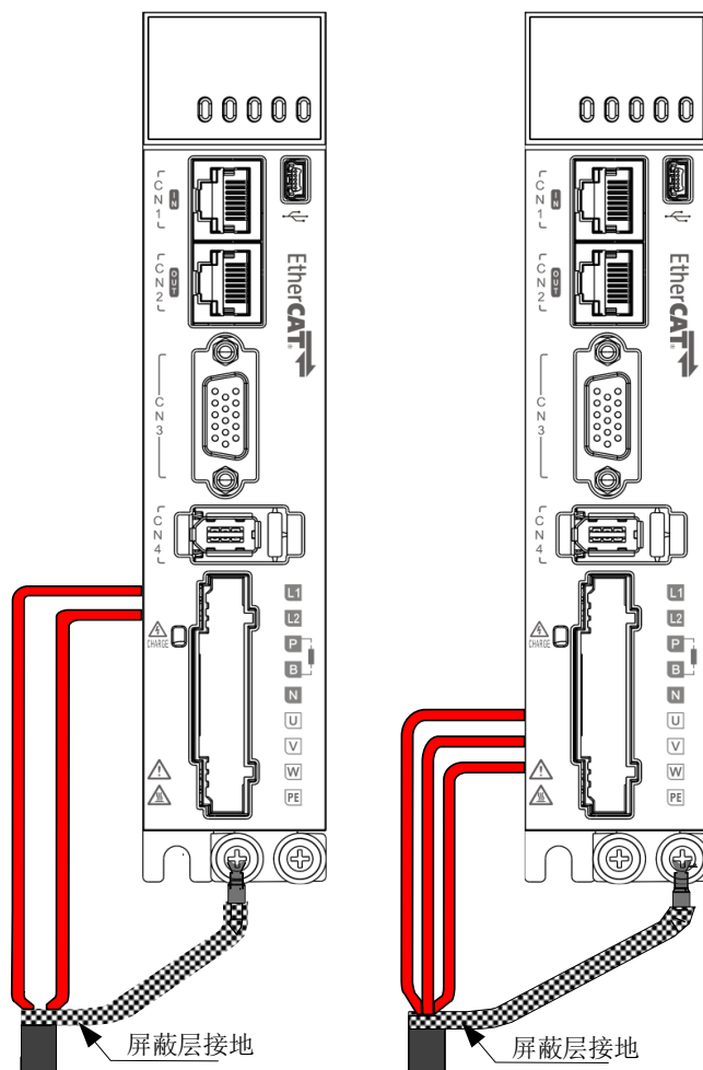
图2-33 输入/输出侧动力线缆屏蔽层接线
