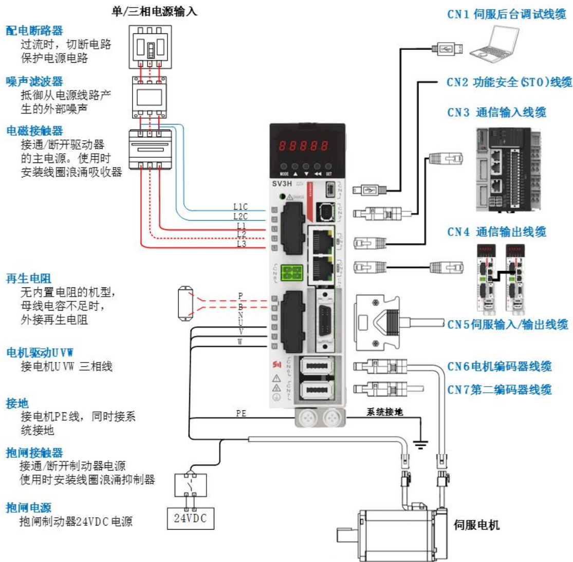
图2-1 SIZE-A 系统配线图
