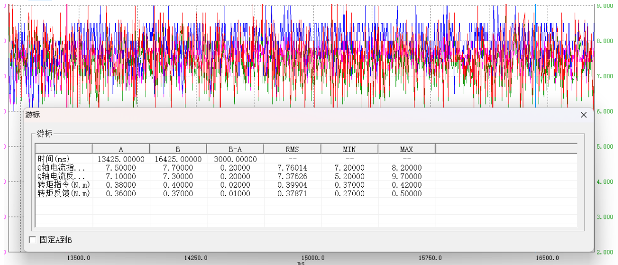
图3-23 游标测量
