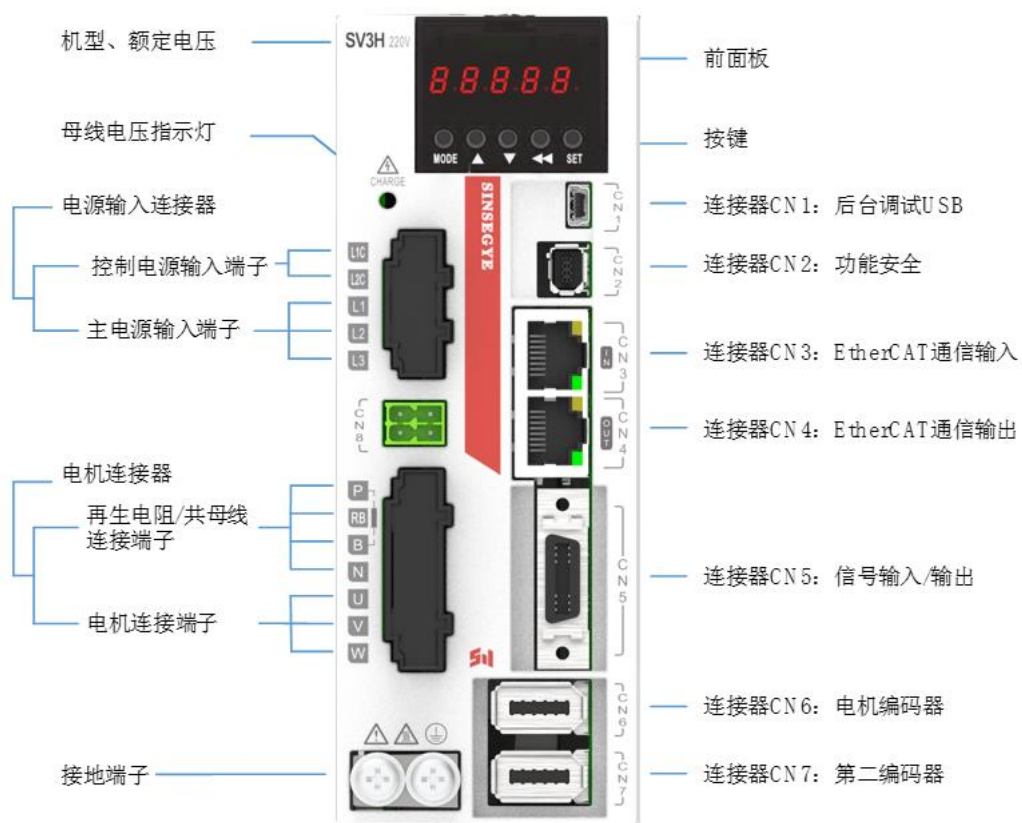
图1-2 SIZE-B 机型接口命名
