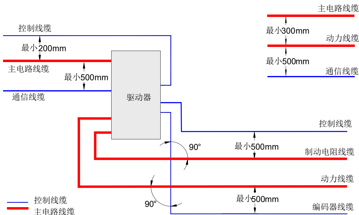
图2-35 推荐的线缆布置图
