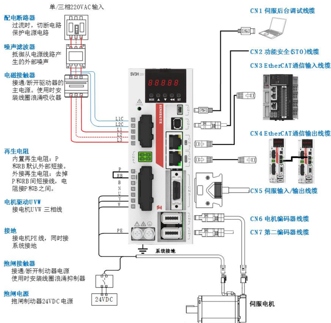
图2-2 SIZE-B 系统配线图
