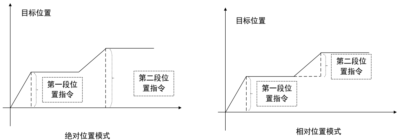
图3-68 PP 模式相对运动与绝对运动区别示意图
