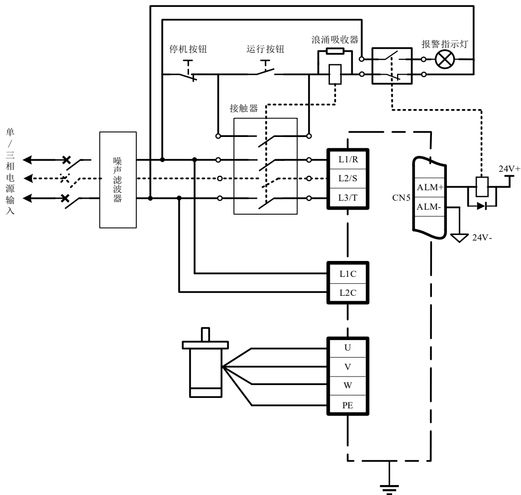
图2-8 SIZE-C 主电路配线示例
