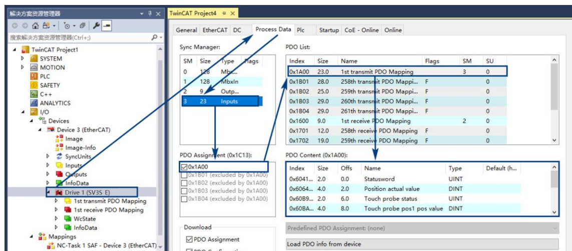
图7-17 TwinCAT3 修改 TPDO 列表
