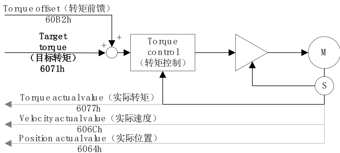
图3-62 同步周期转矩模式 (CST) 概览图
