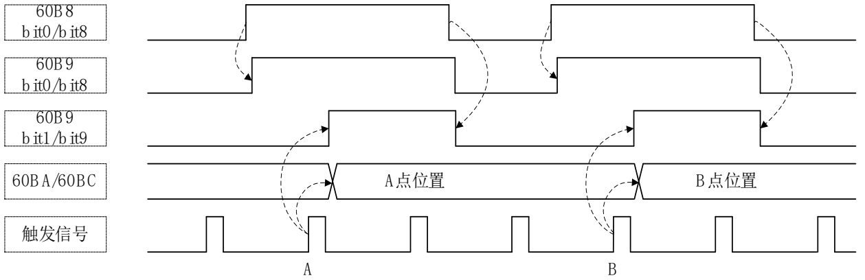
图3-76 单次上升沿锁存示意图
