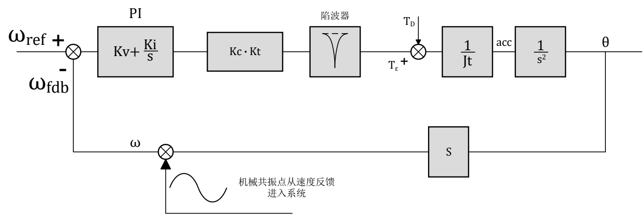
图4-20 共振抑制控制框图
