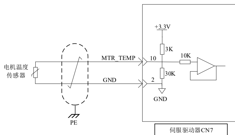
图2-24 电机温度传感器接线图
