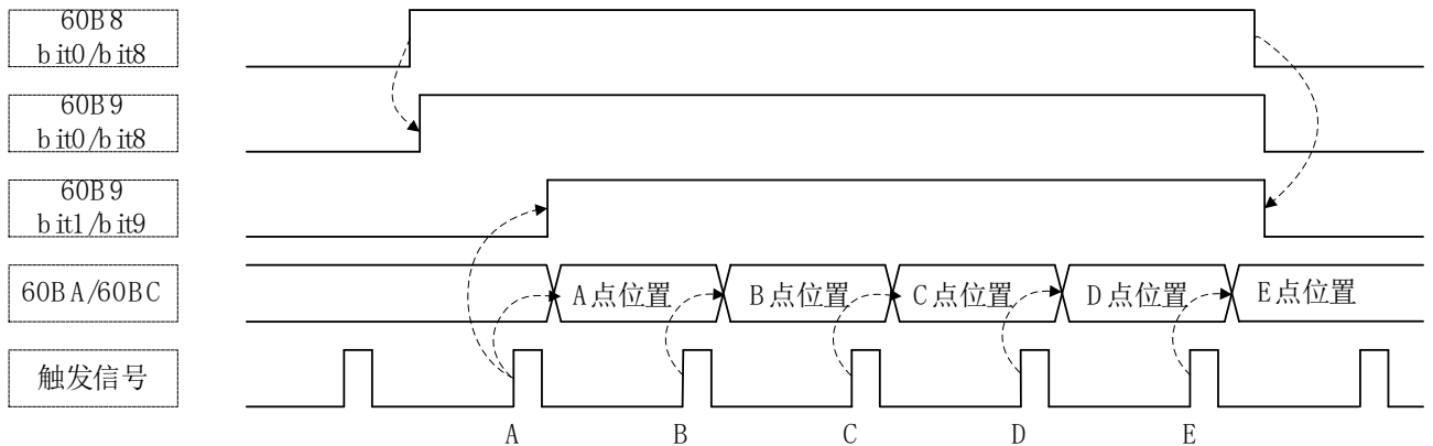
图3-78 连续上升沿锁存
