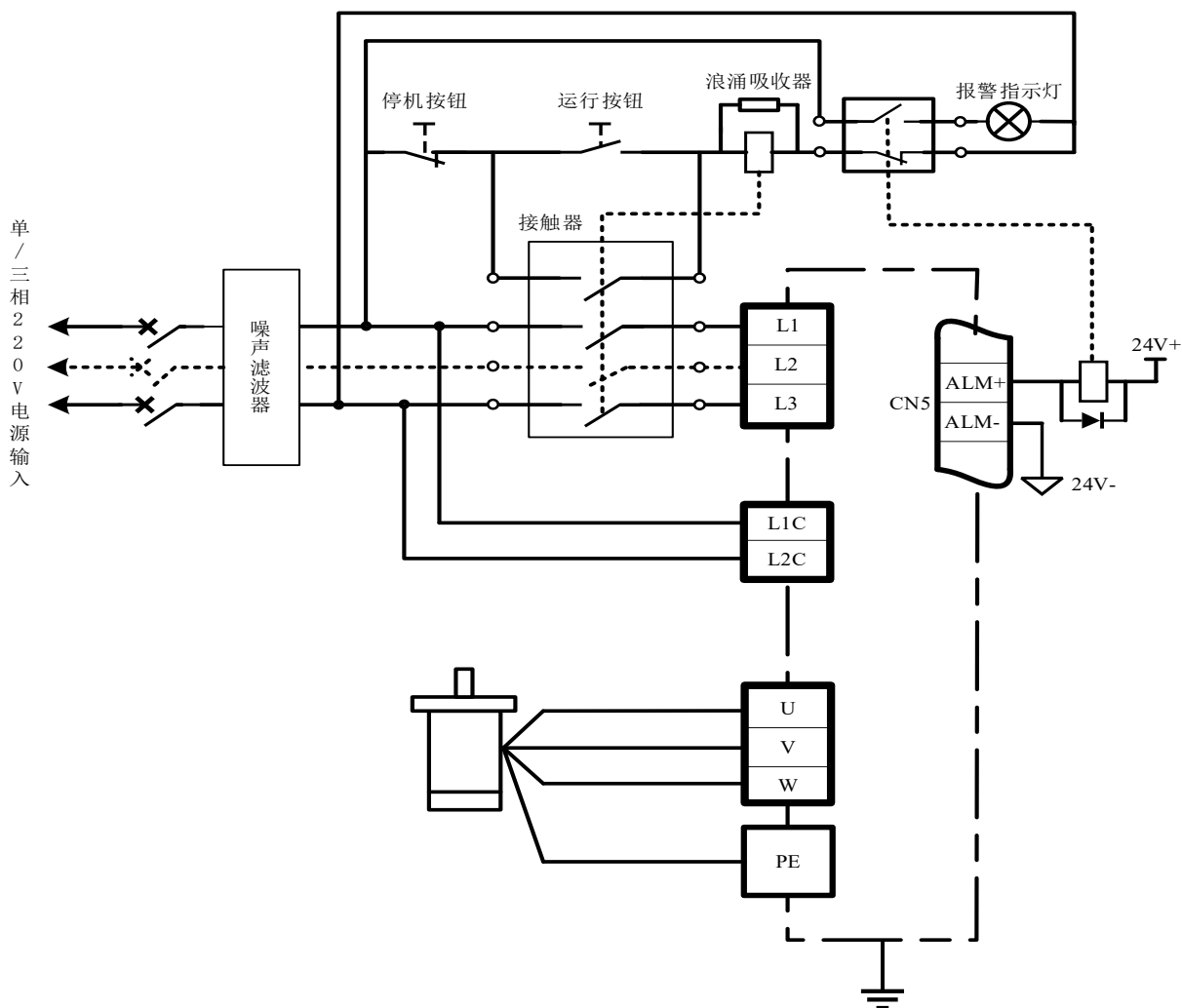
图2-6 SIZE-A 主电路配线示例
