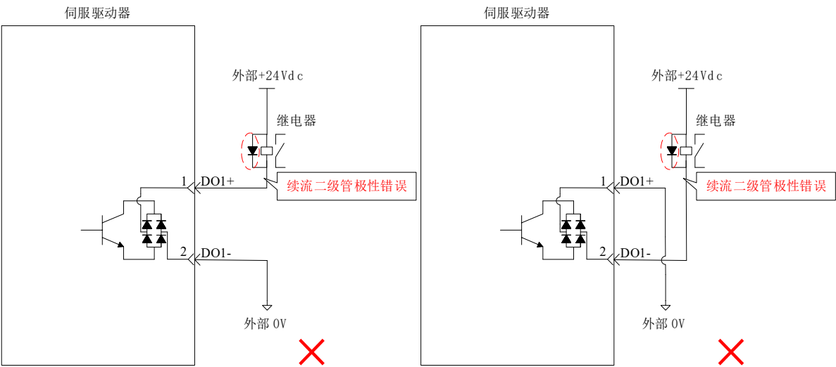
图2-18 数字量输出接线示意图（继电器输入，错误接线）
