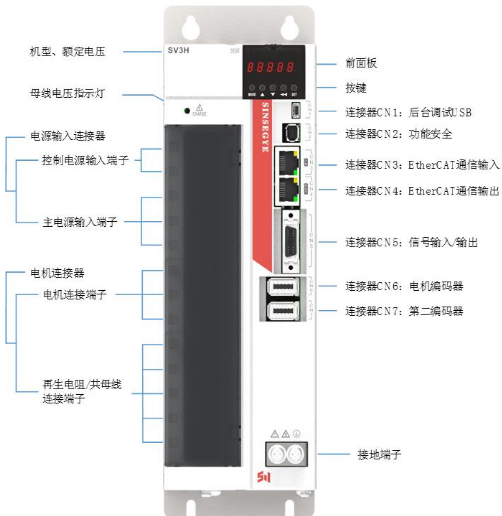
图1-4 SIZE-D 机型接口命名
