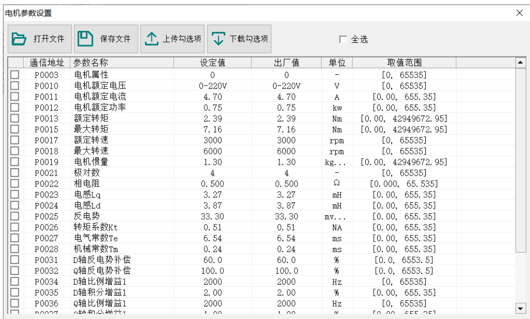
图3-27 电机参数管理
