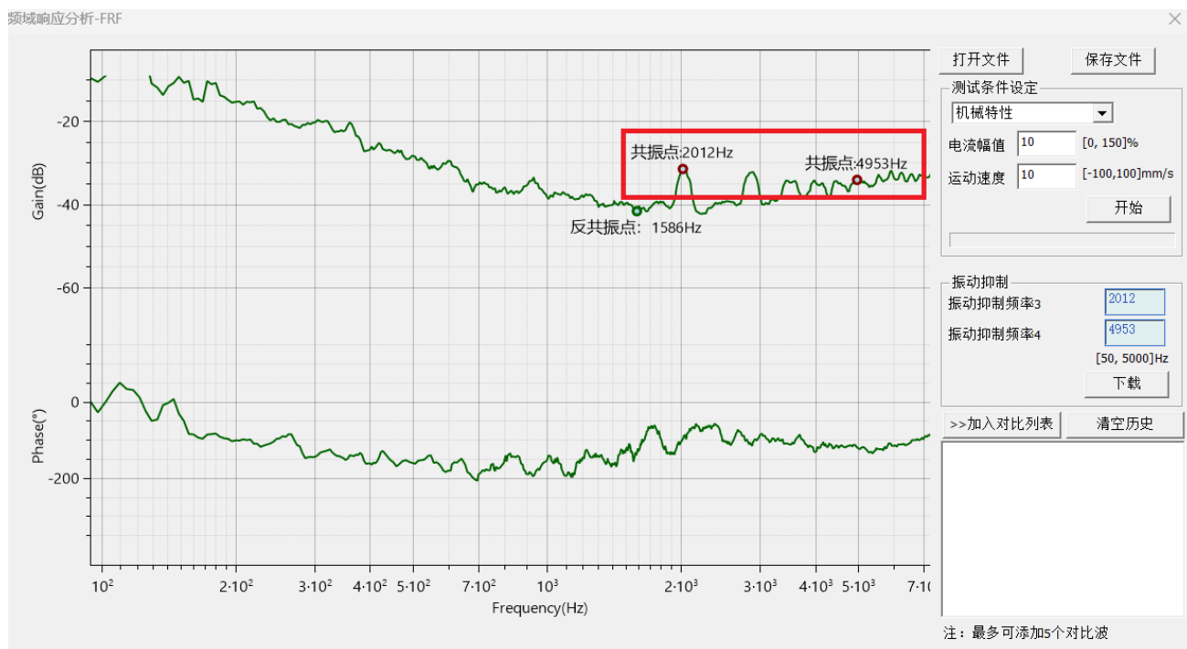
图3-47 机械特性
