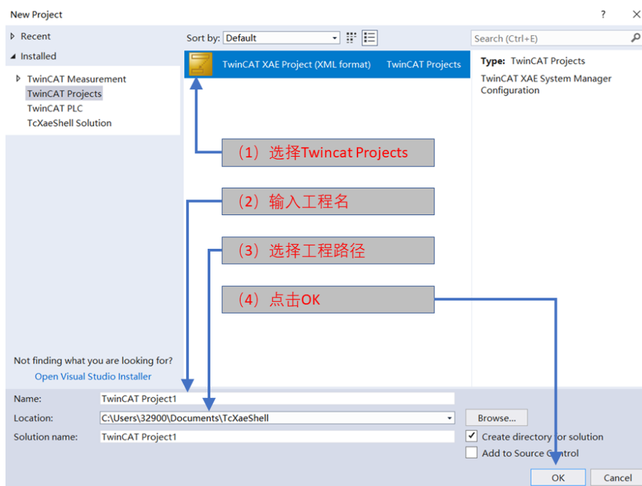
图7-4 TwinCAT 新建工程界面
