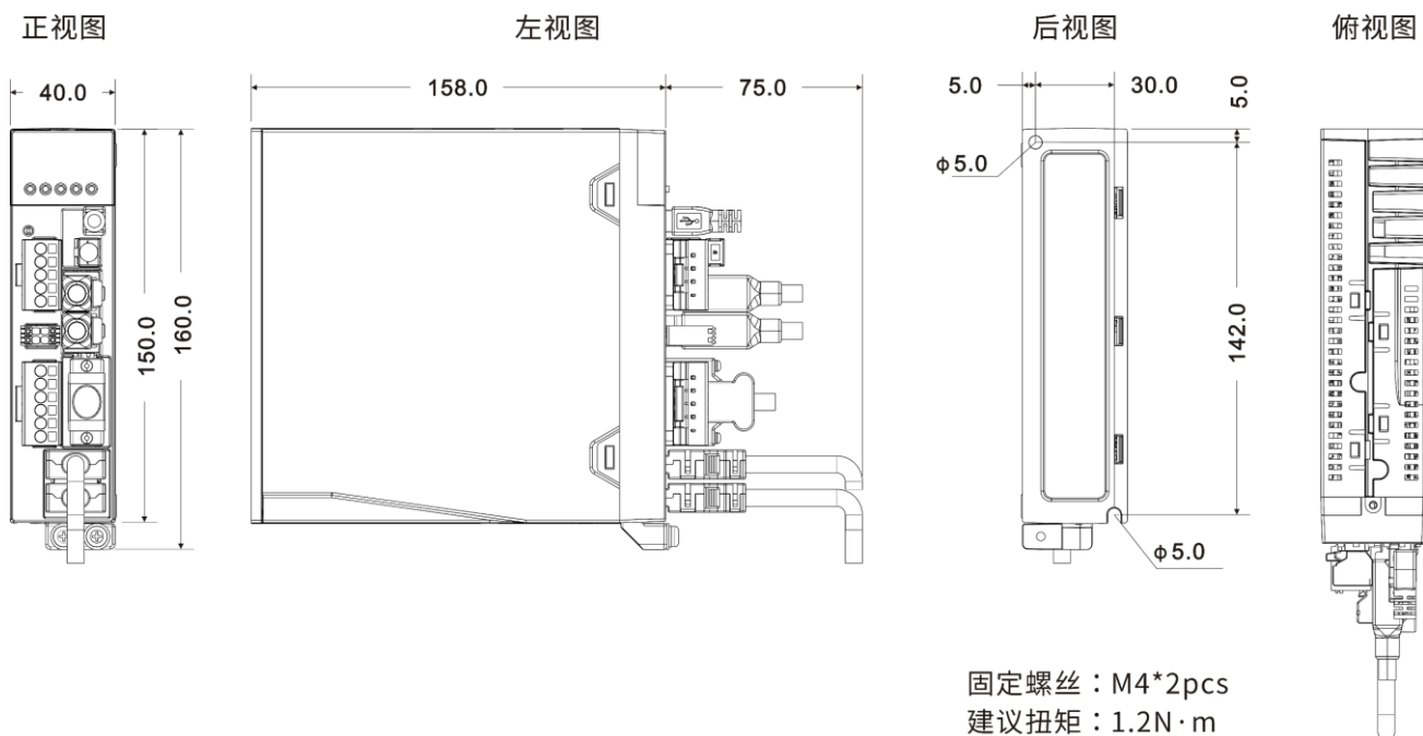
图1-5 SIZE-A 外形尺寸图（单位 mm）
