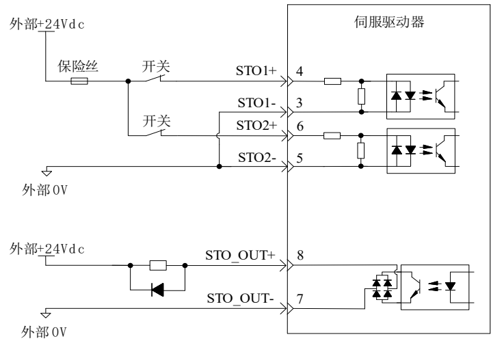
图2-26 功能安全接线说明
