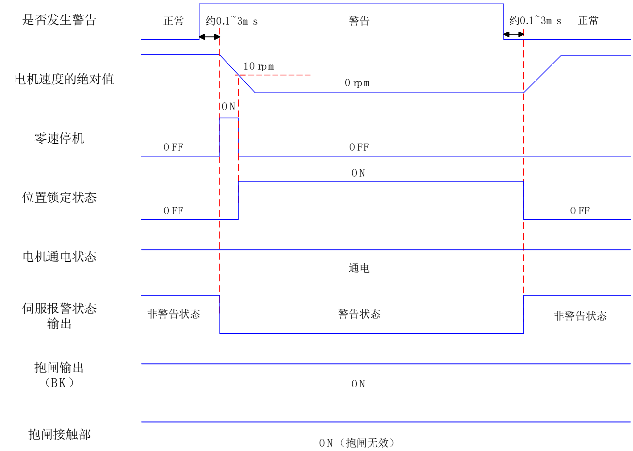
图3-12 需停机类警告时序图
