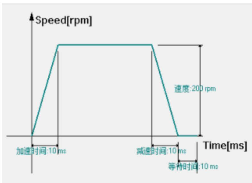
图3-36 运行轨迹生成
