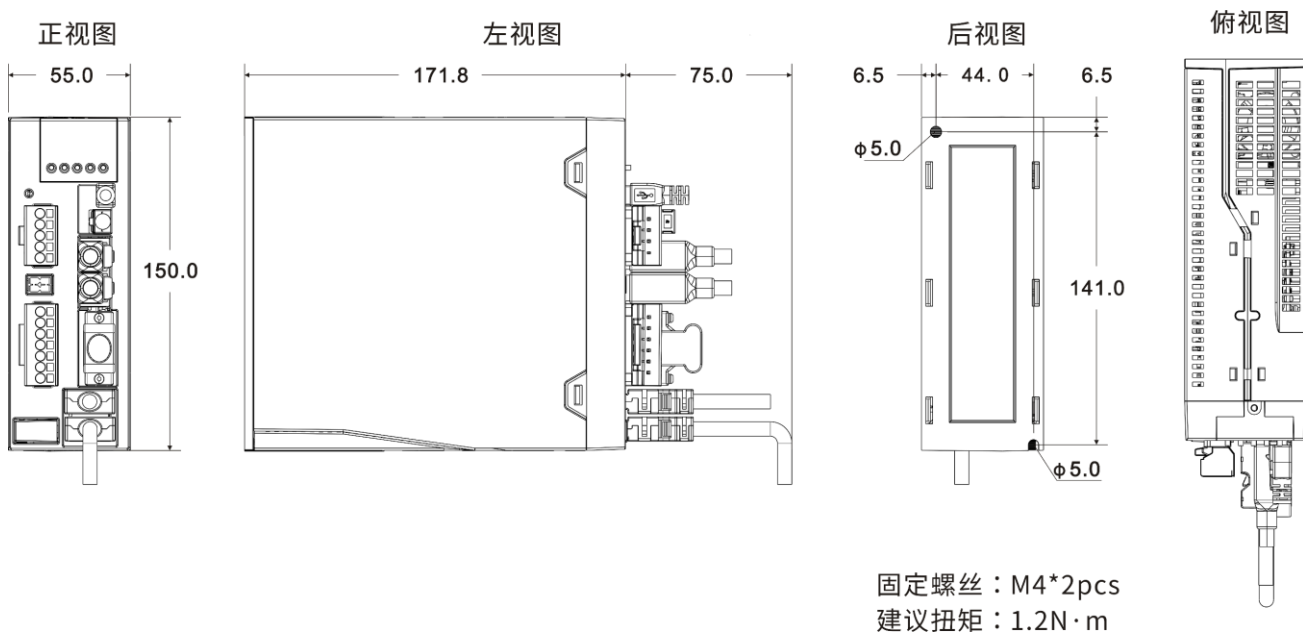
图1-6 SIZE-B 外形尺寸图（单位 mm）
