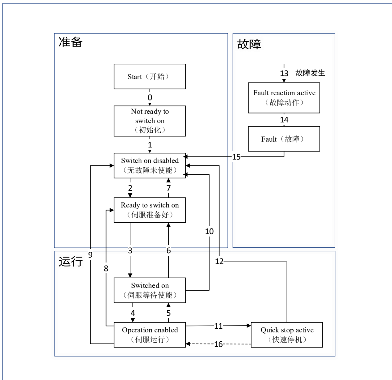
图3-52 CiA402 状态机切换图
