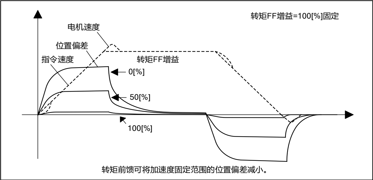
图4-15 转矩前馈增益与加减速段位置偏差大小关系
