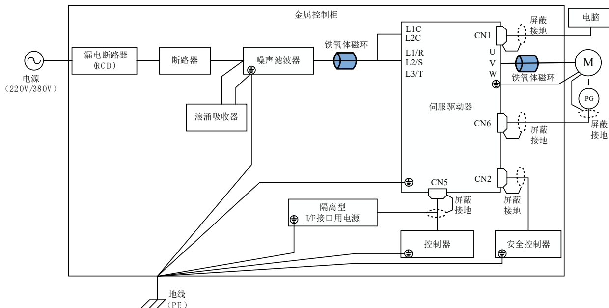
图2-27 伺服驱动器抗干扰措施示意图
