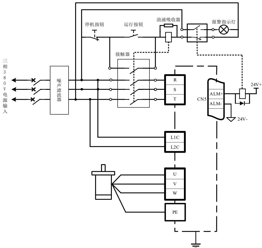
图2-9 SIZE-D 主电路配线示例
