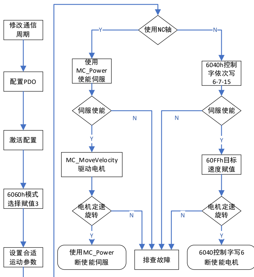
图7-25 PV 模式使用示例流程图
