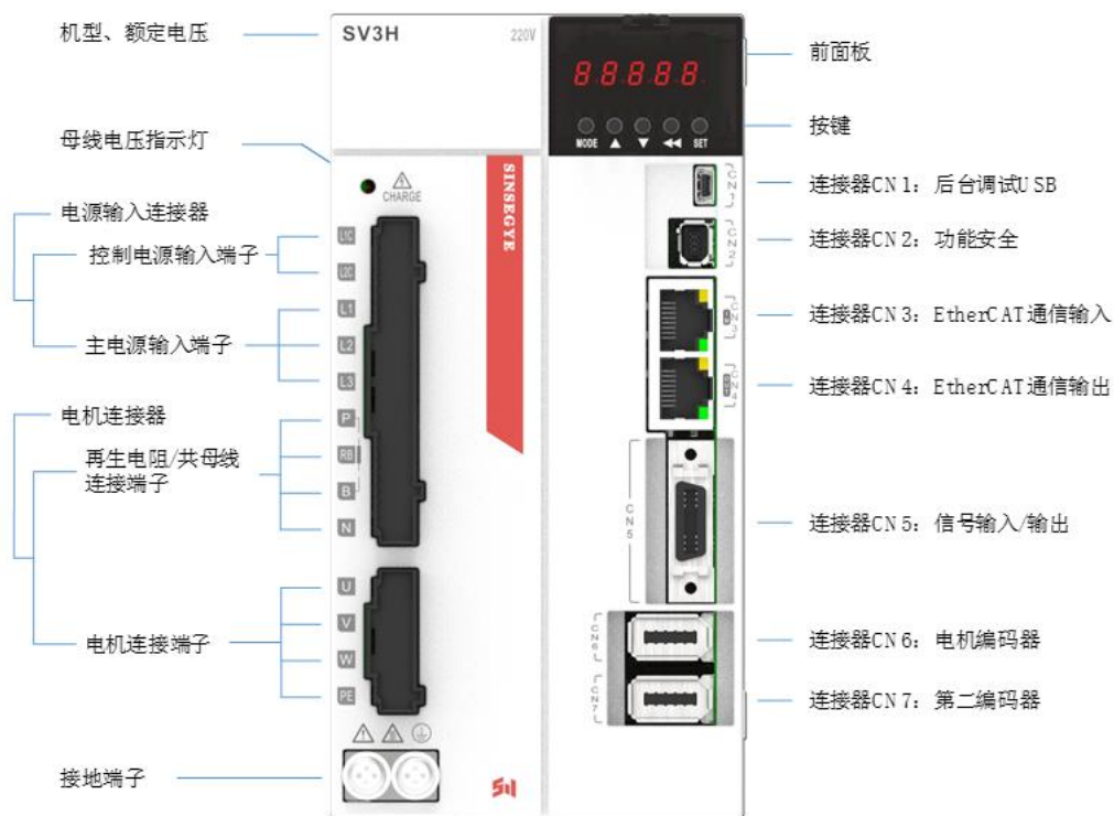
图1-3 SIZE-C 机型接口命名
