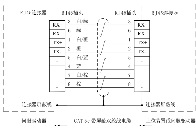
图2-25 EtherCAT 通讯接线说明
