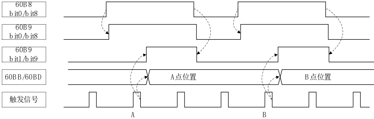
图3-77 单次下降沿锁存示意图
