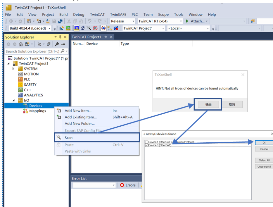
图7-6 TwinCAT3 扫描设备
