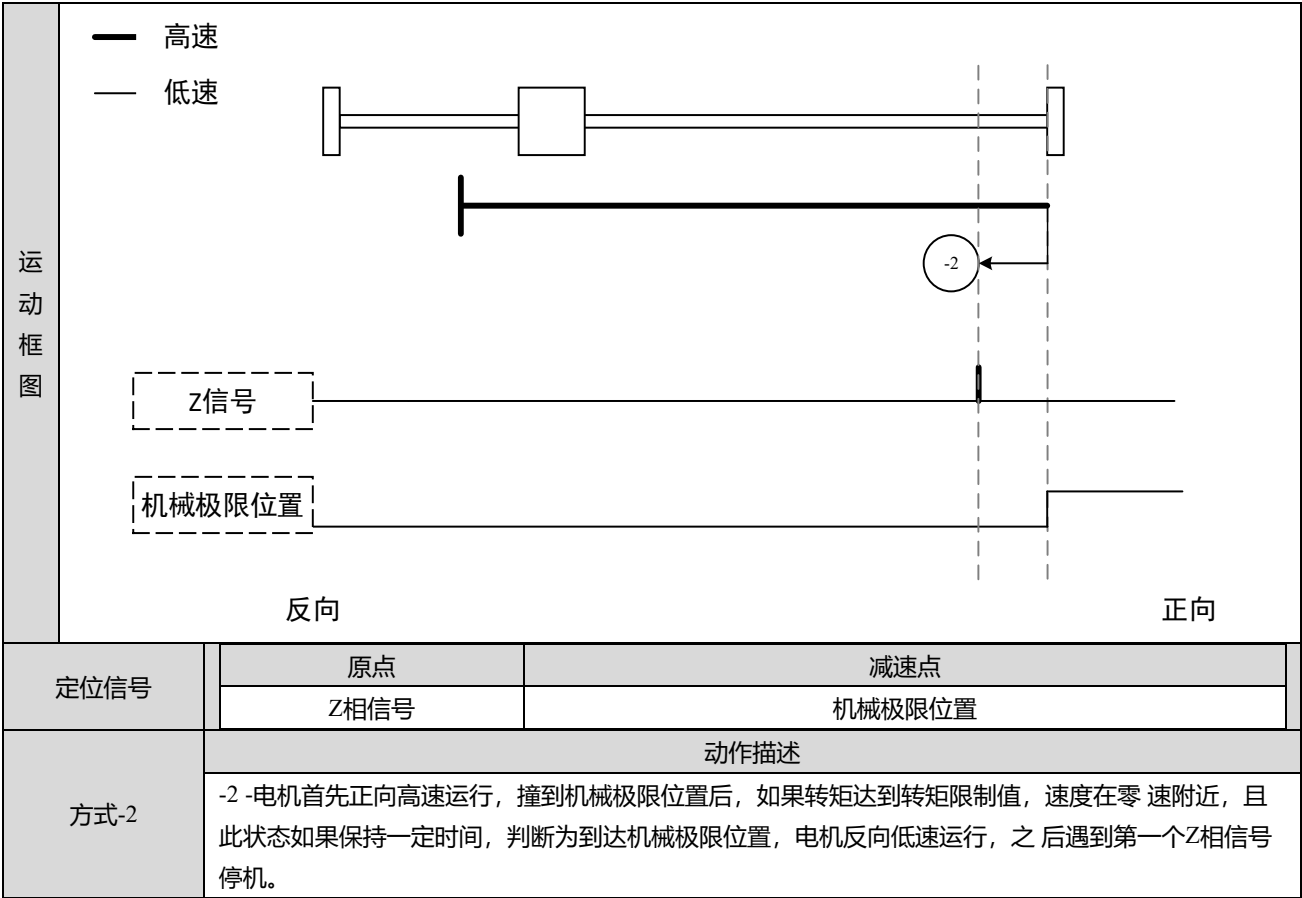
图3-75 原点复归模式 -2
