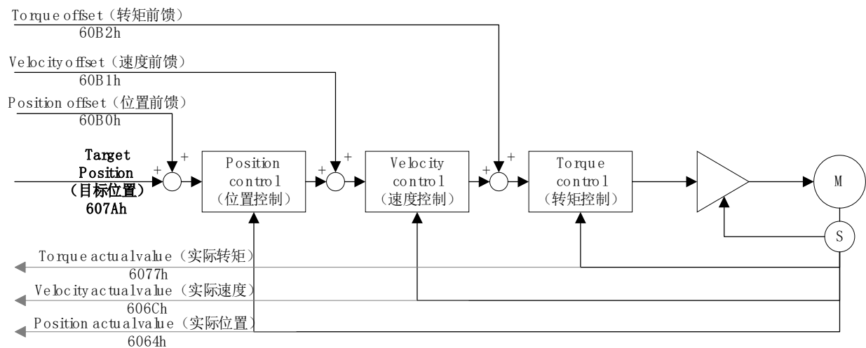
图3-53 同步周期位置模式概览图
