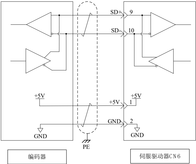
图2-22 电机编码器信号输入
