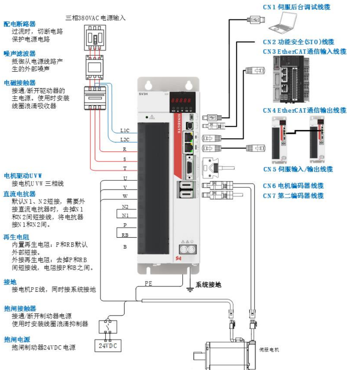
图2-4 SIZE-D 系统配线图
