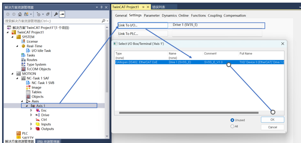
图7-10 链接 NC 轴与物理轴
