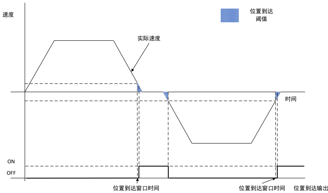
图3-56 CSP 模式定位完成功能示意图
