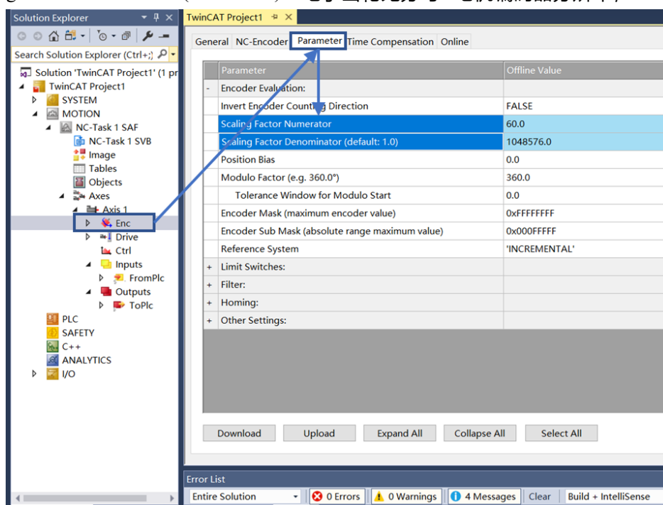
图7-11 修改 NC 轴电子齿轮比
