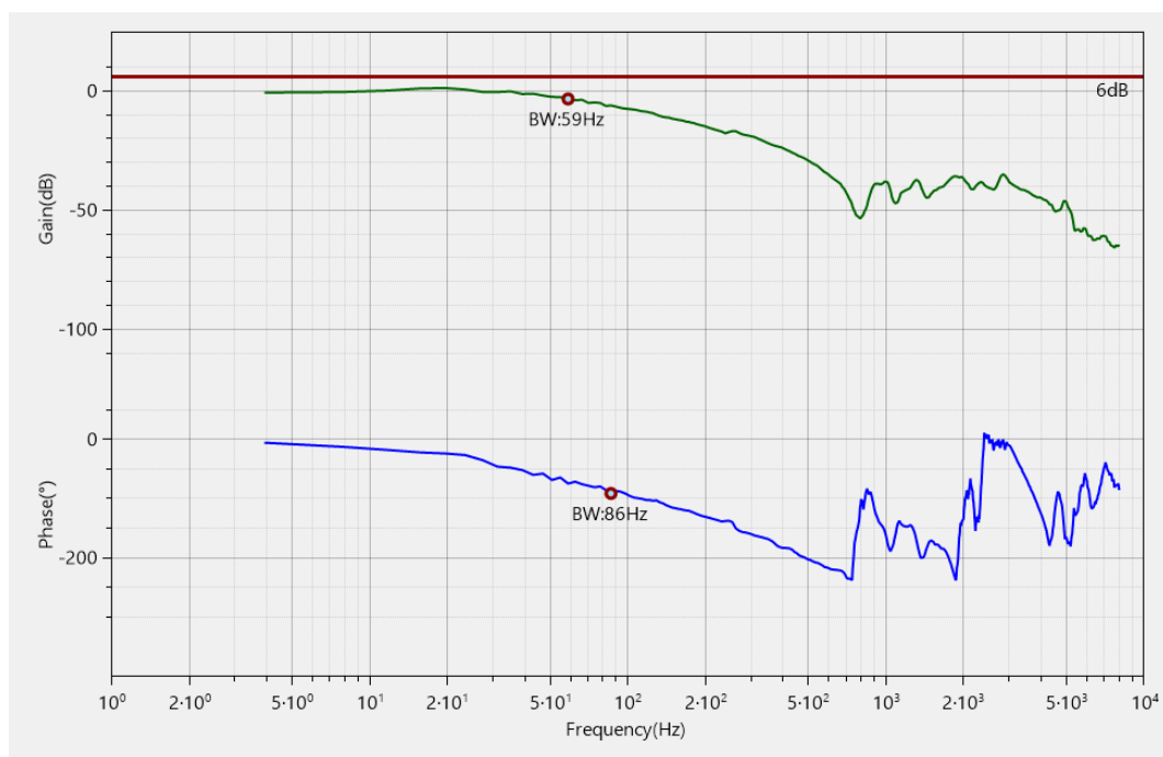
图3-45 速度闭环
