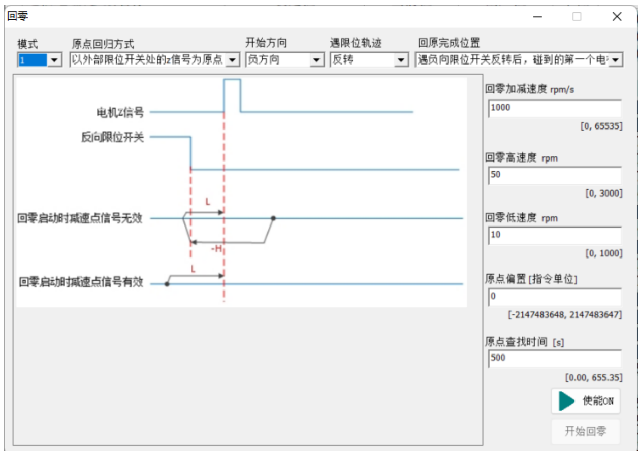
图3-41 回零
