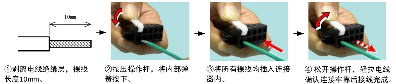
图2-5 卡簧式端子接线方法
