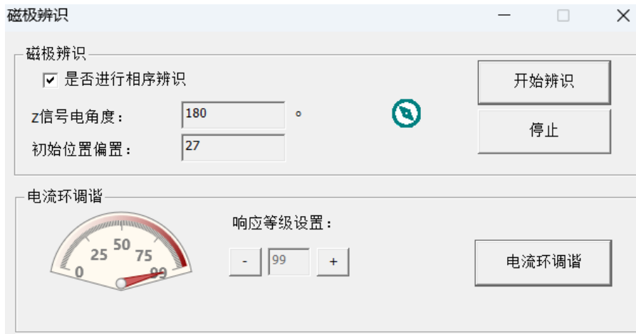
图3-29 磁极辨识
