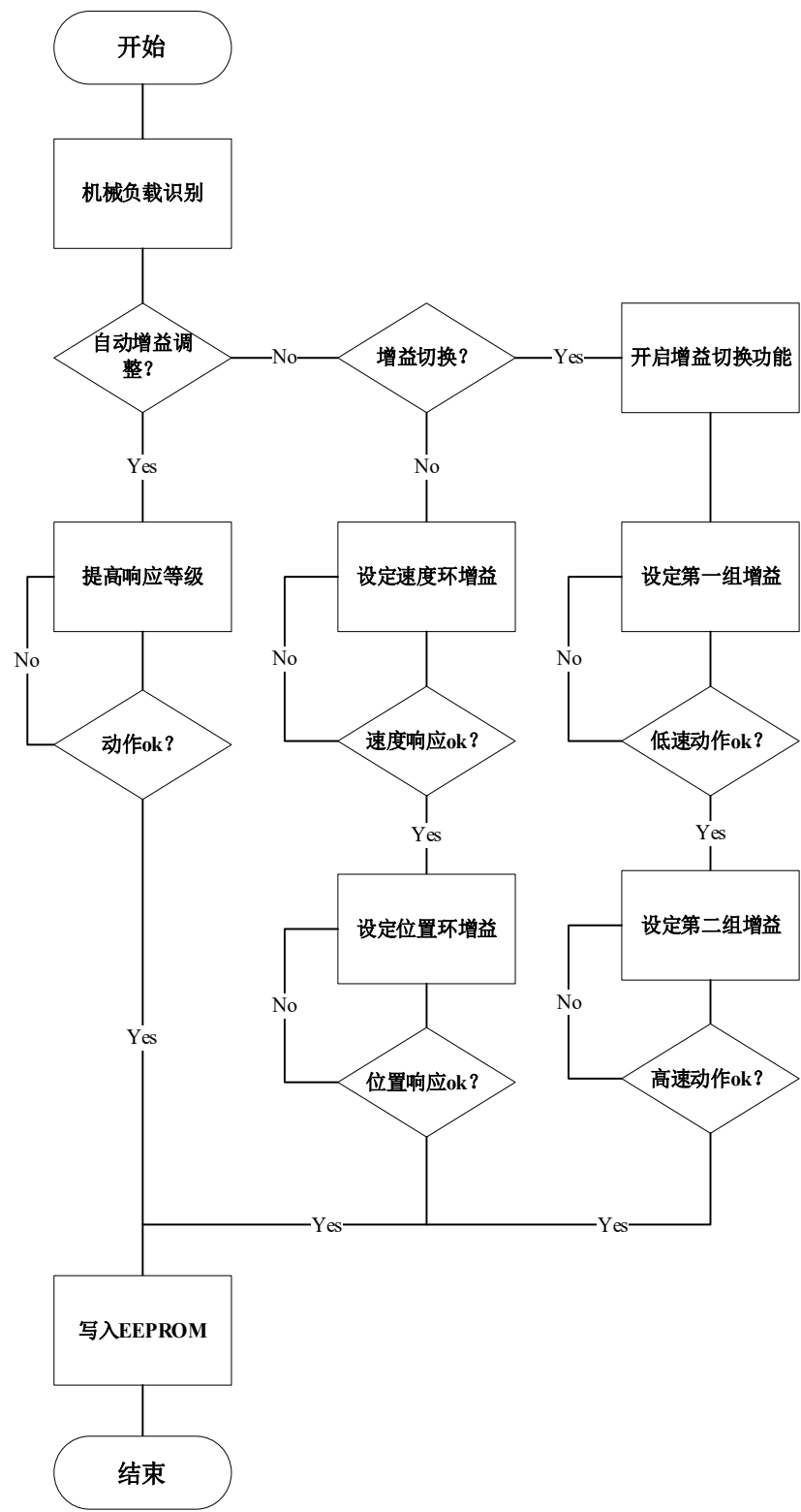
图4-2 增益调整流程
