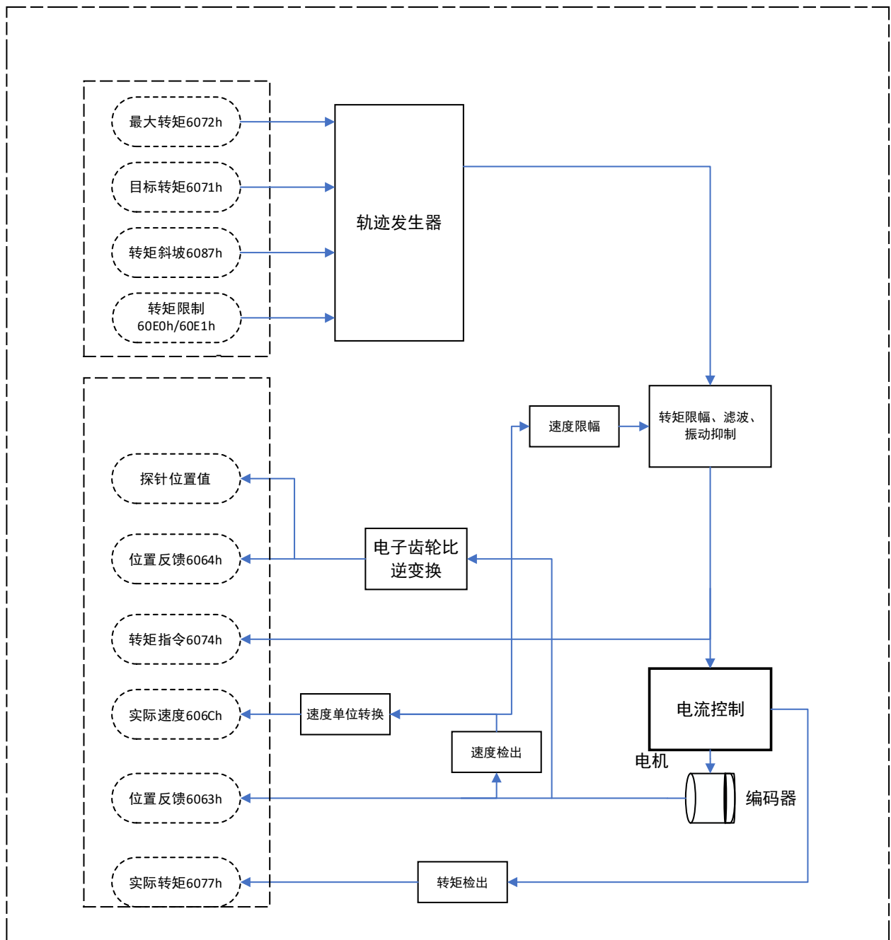
图3-71 轮廓转矩模式 (PT) 控制框图
