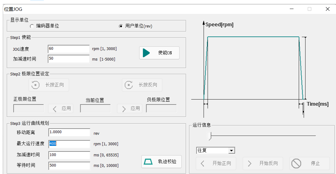
图3-32 位置 JOG
