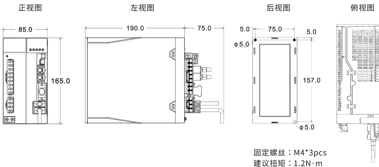
图1-7 SIZE-C 外形尺寸图 (单位 mm)
