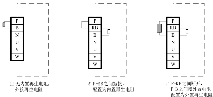
图2-11 再生电阻接线
