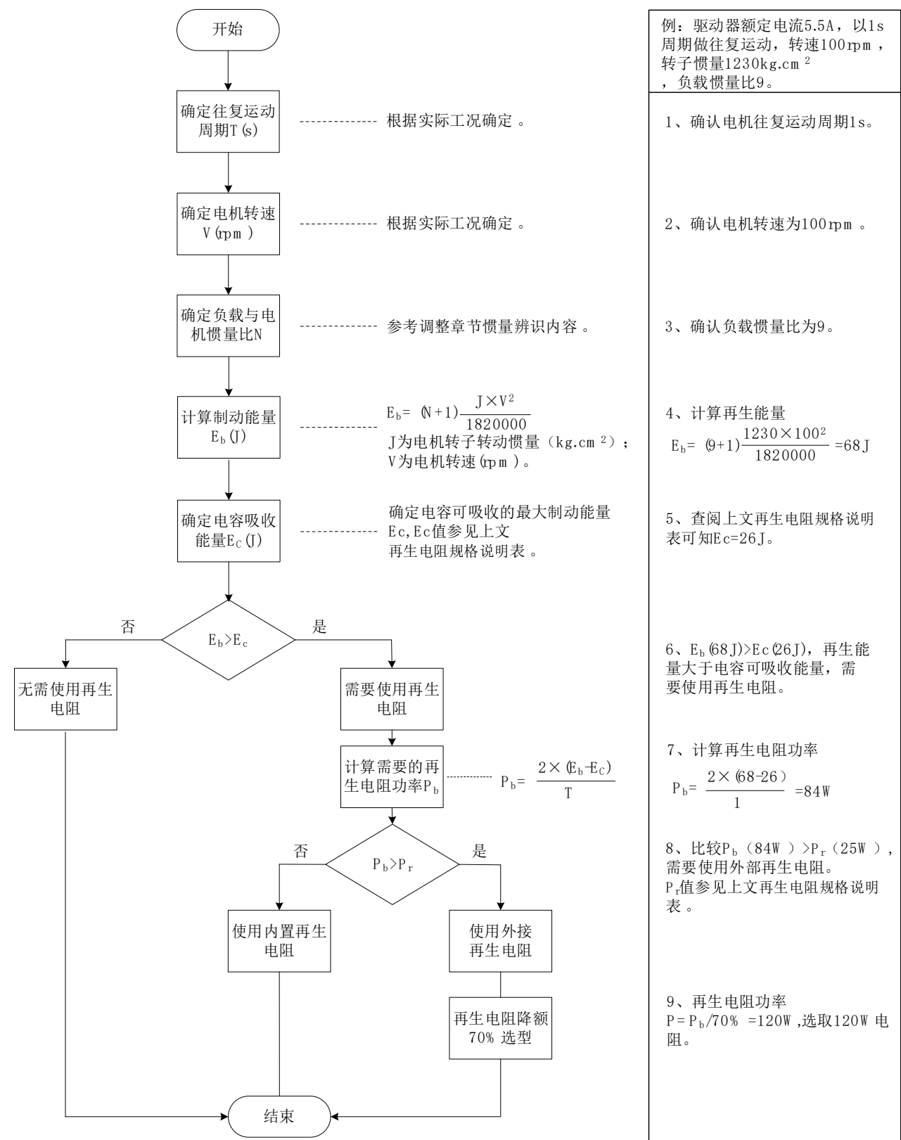
图2-12 再生电阻选型流程
