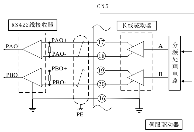
图2-21 分频输出接线
