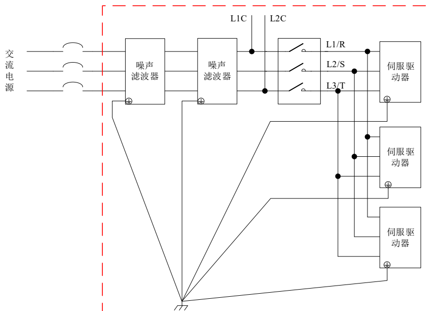
图2-28 噪声滤波器串联使用安装与接地示意图
