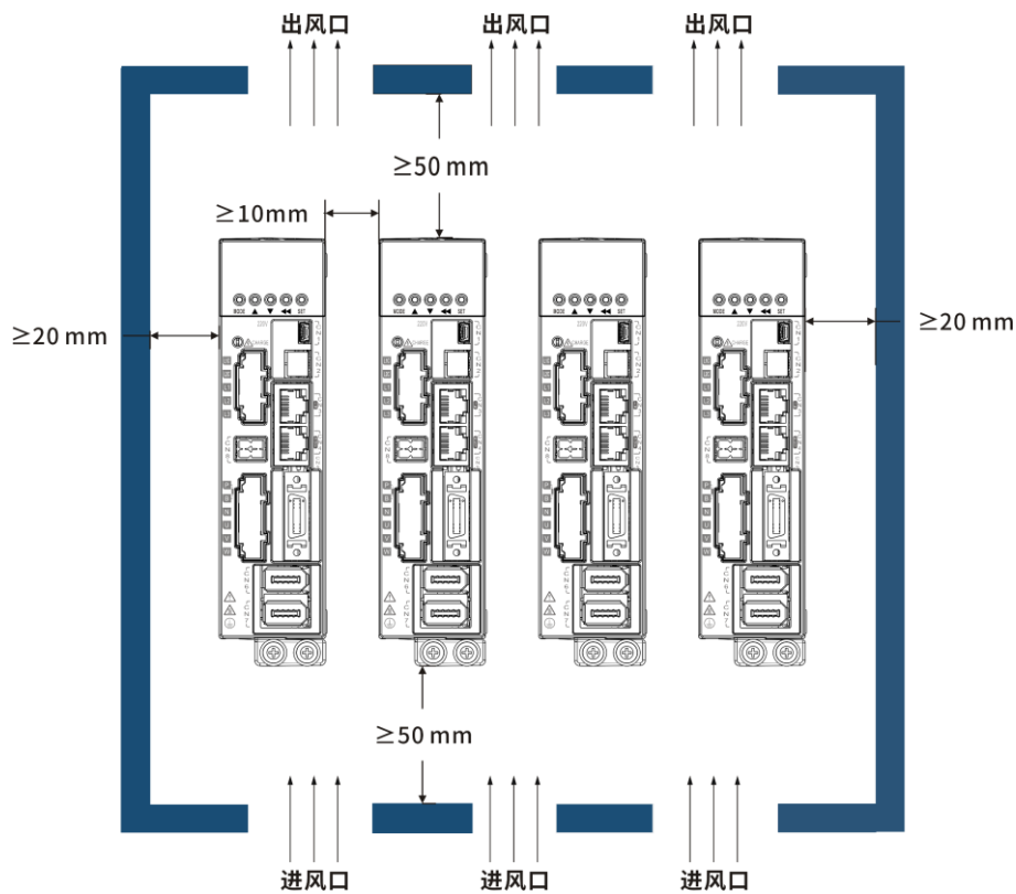
图1-9 伺服驱动器安装示意图（保留间距安装时）
