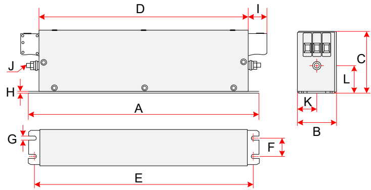
图2-31 FN3258 系列 7-30A 滤波器尺寸图(单位: mm)
