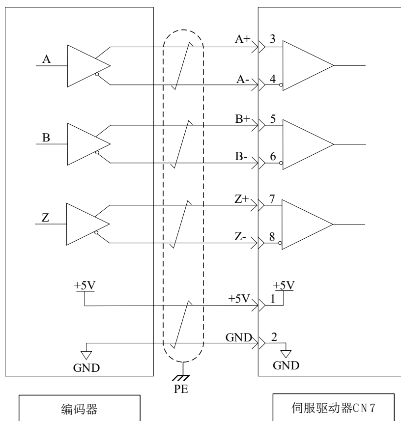
图2-23 第二编码器差分信号输入
