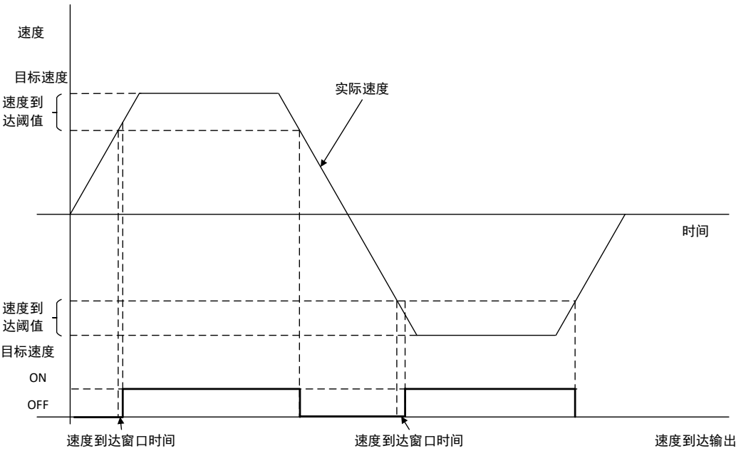
图3-70 PV 模式速度达到示意图
