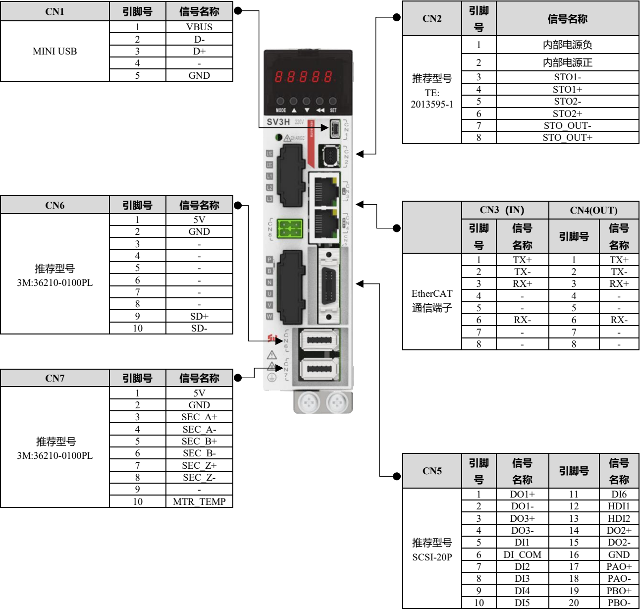
驱动器控制信号端口定义
