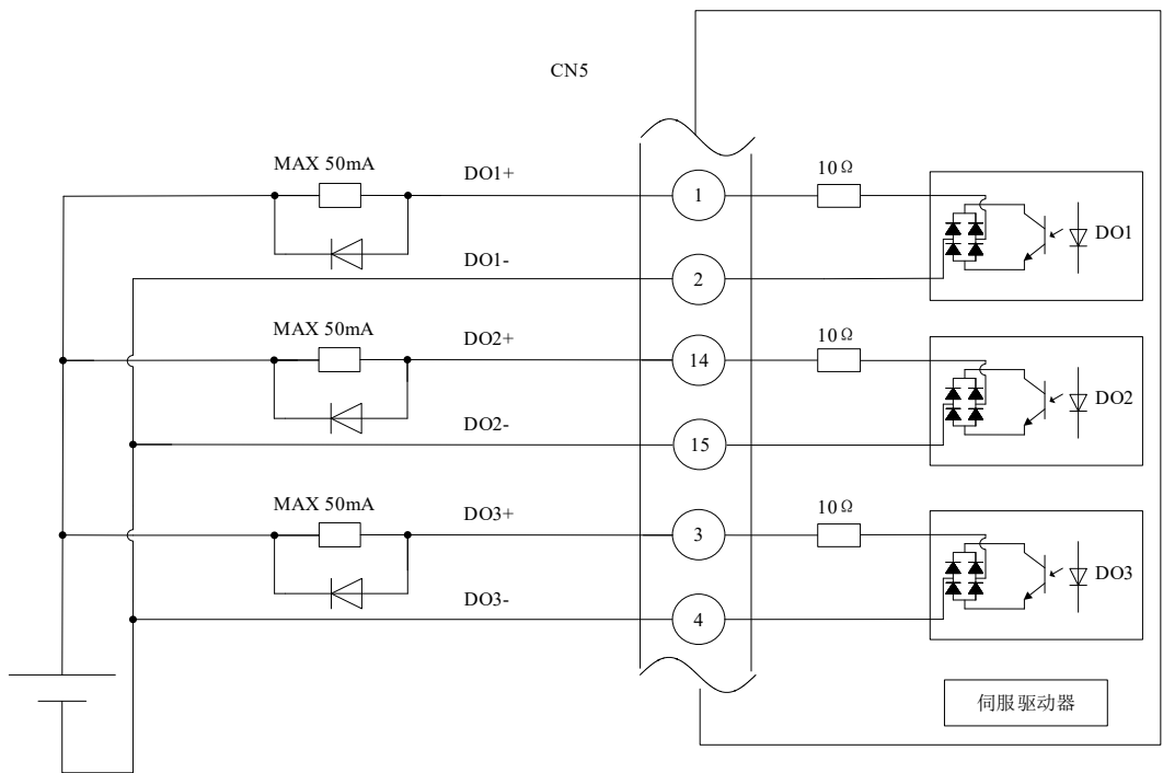
图2-16 数字量输出接线
