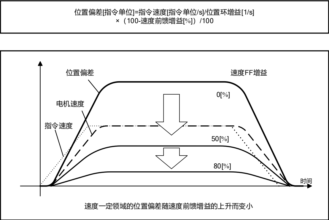
图4-13 速度前馈增益与位置偏差关系
