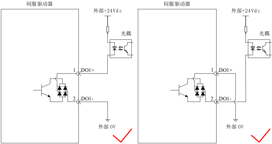
图2-19 数字量输出接线示意图（光耦输入，正确接线）
