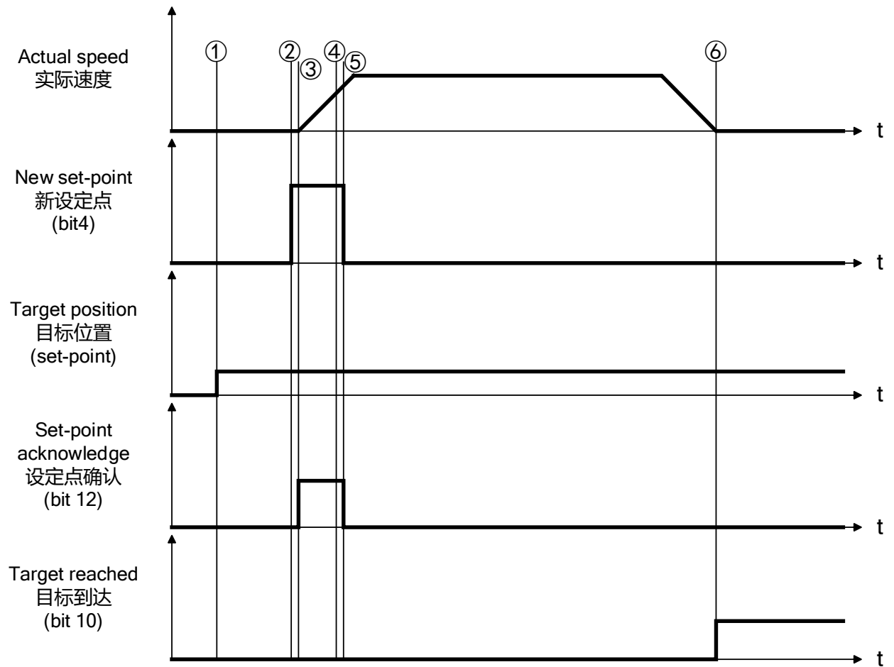
图3-65 PP 模式基本 set-point
