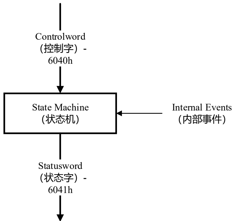
图3-51 Cia402 协议概览图
