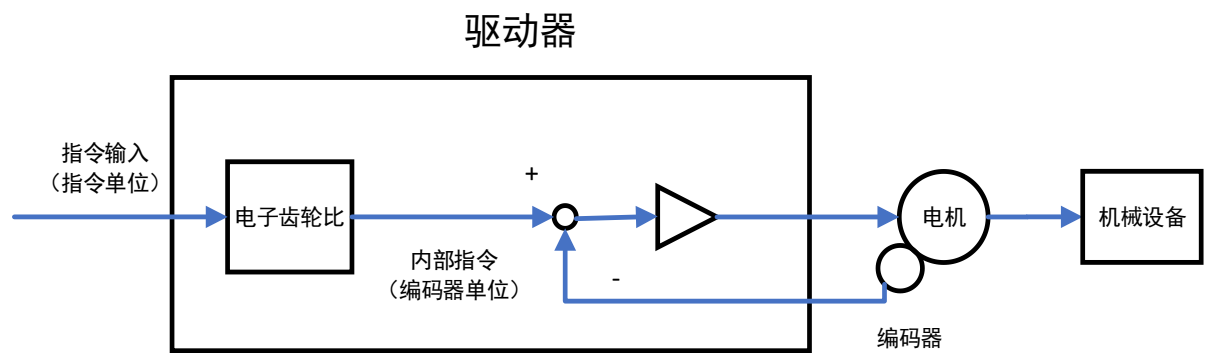
图3-5 电子齿轮比
