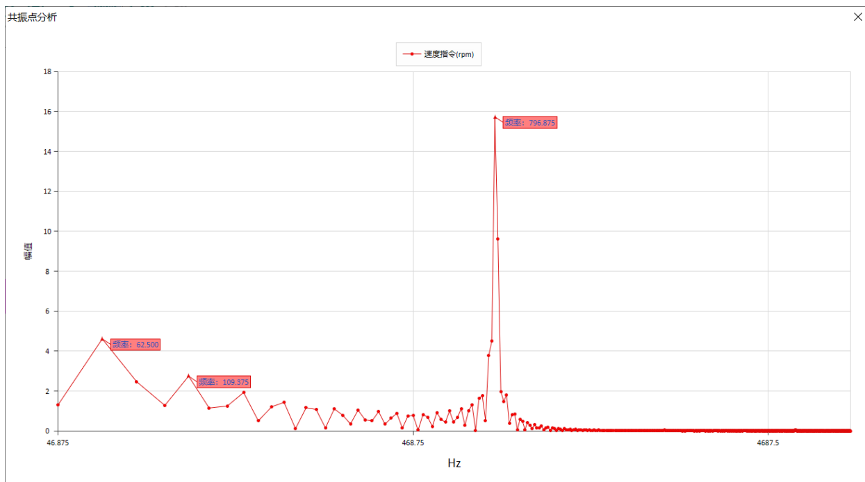
图3-24 FFT 共振点分析
