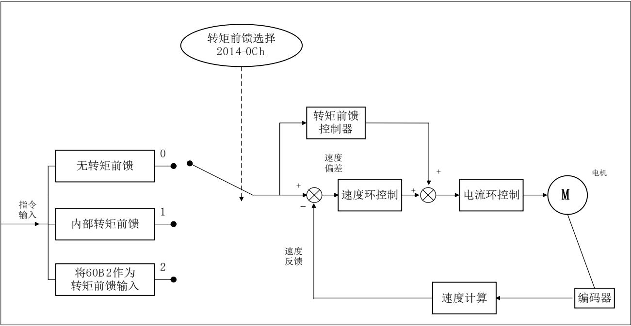
图4-14 转矩前馈控制操作图
