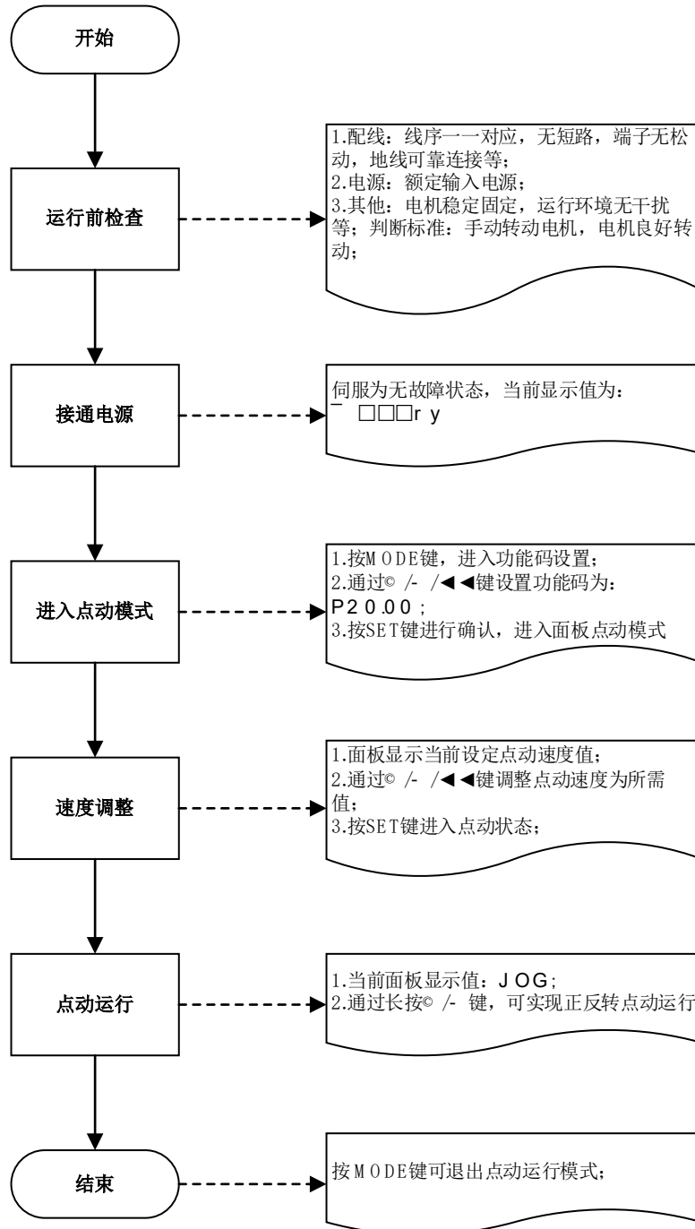
图3-17 面板点动运行操作流程
