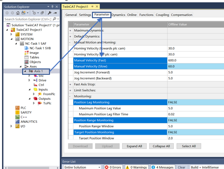
图7-12 NC 轴点动高速与低速设置
