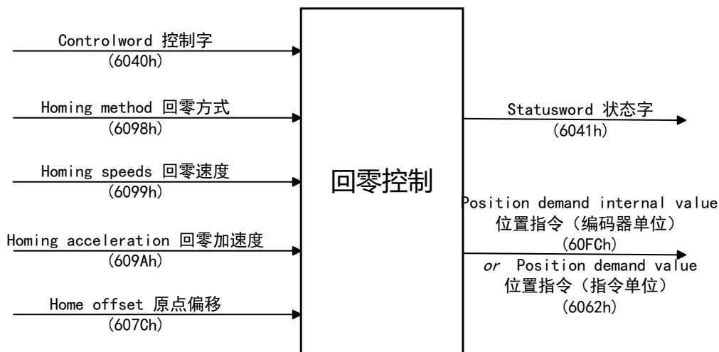
图3-72 回零模式控制框图
