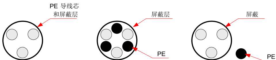
图2-32 推荐的动力电缆类型
