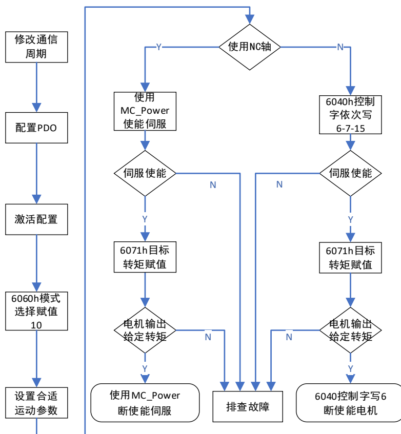
图7-23 CST 模式使用示例流程图
