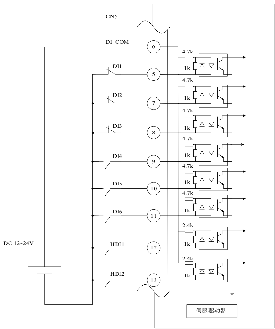
图2-13 数字量输入接线
