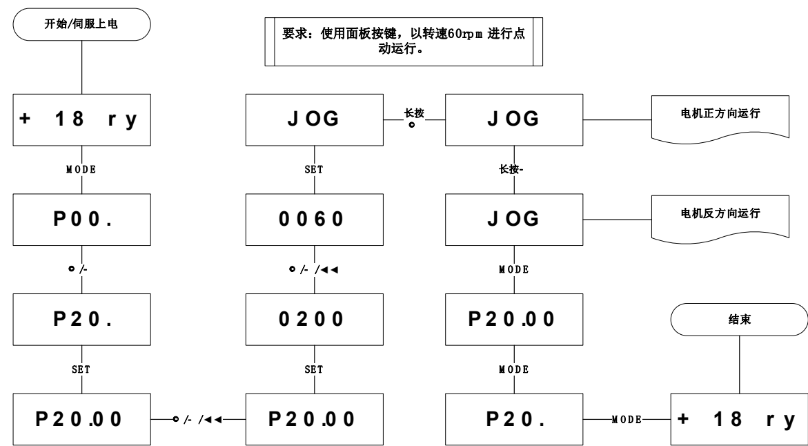
图3-16 面板点动运行示例操作与显示图
