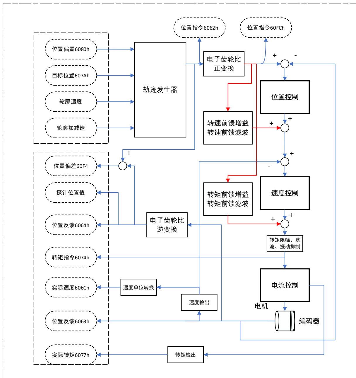
图3-64 轮廓位置模式框图
