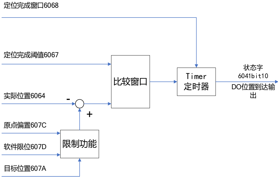
图3-55 CSP 定位完成概览图
