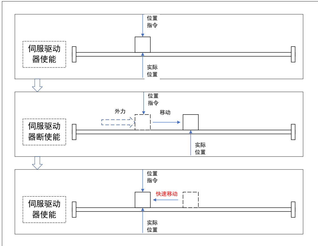
图3-58 CSP 位置对齐示例图
