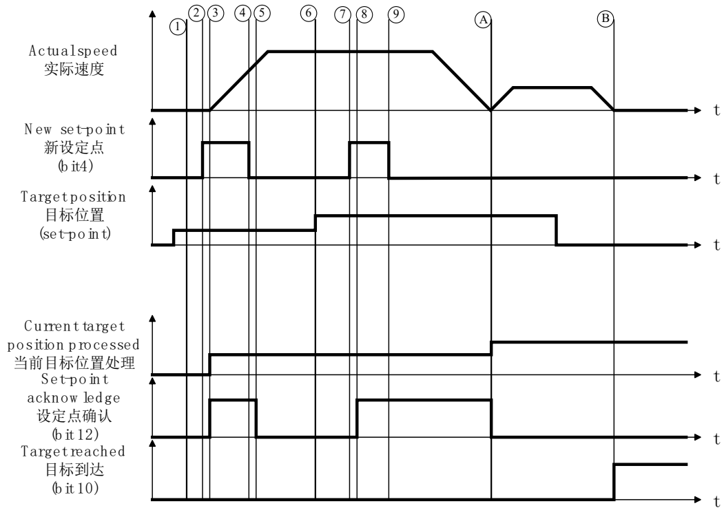
图3-66 PP 模式 set of set-point (非立即更新模式)
