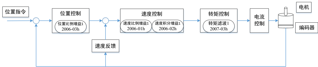
图4-6 手动增益基本说明框图
