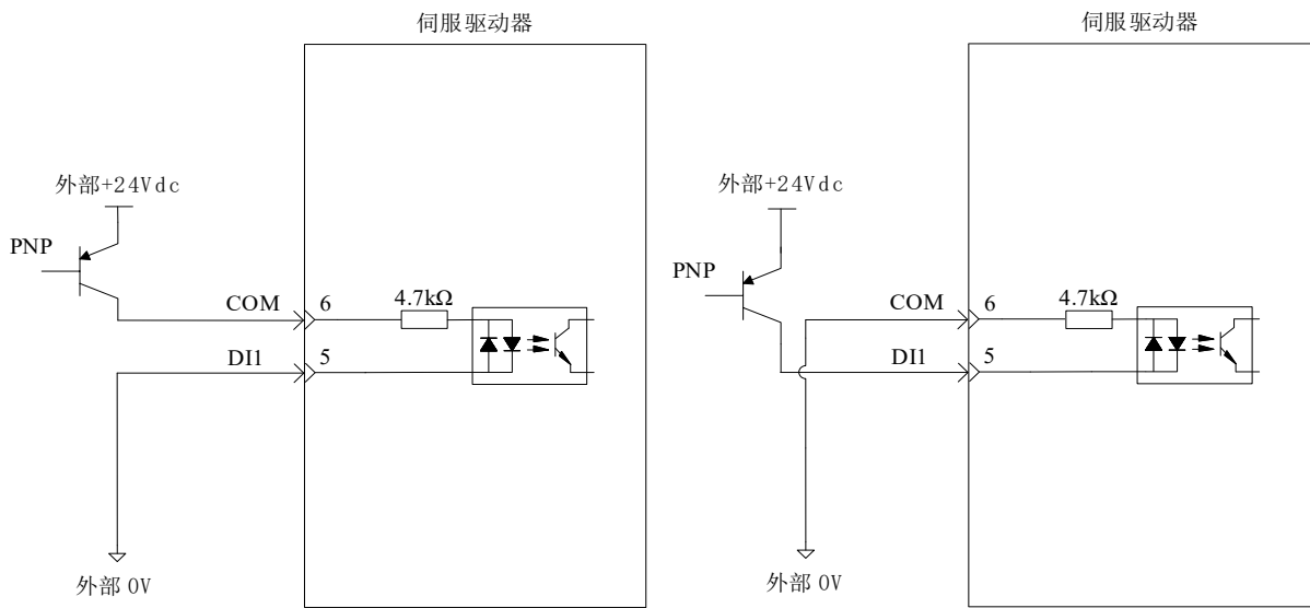
图2-15 数字输入接线示意图（集电极开路）
