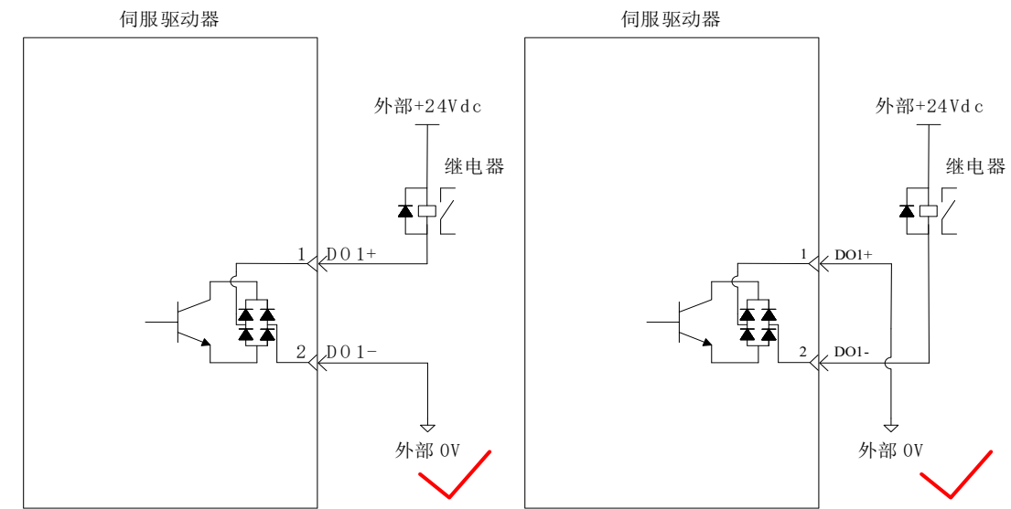
图2-17 数字量输出接线示意图（继电器输入，正确接线）
