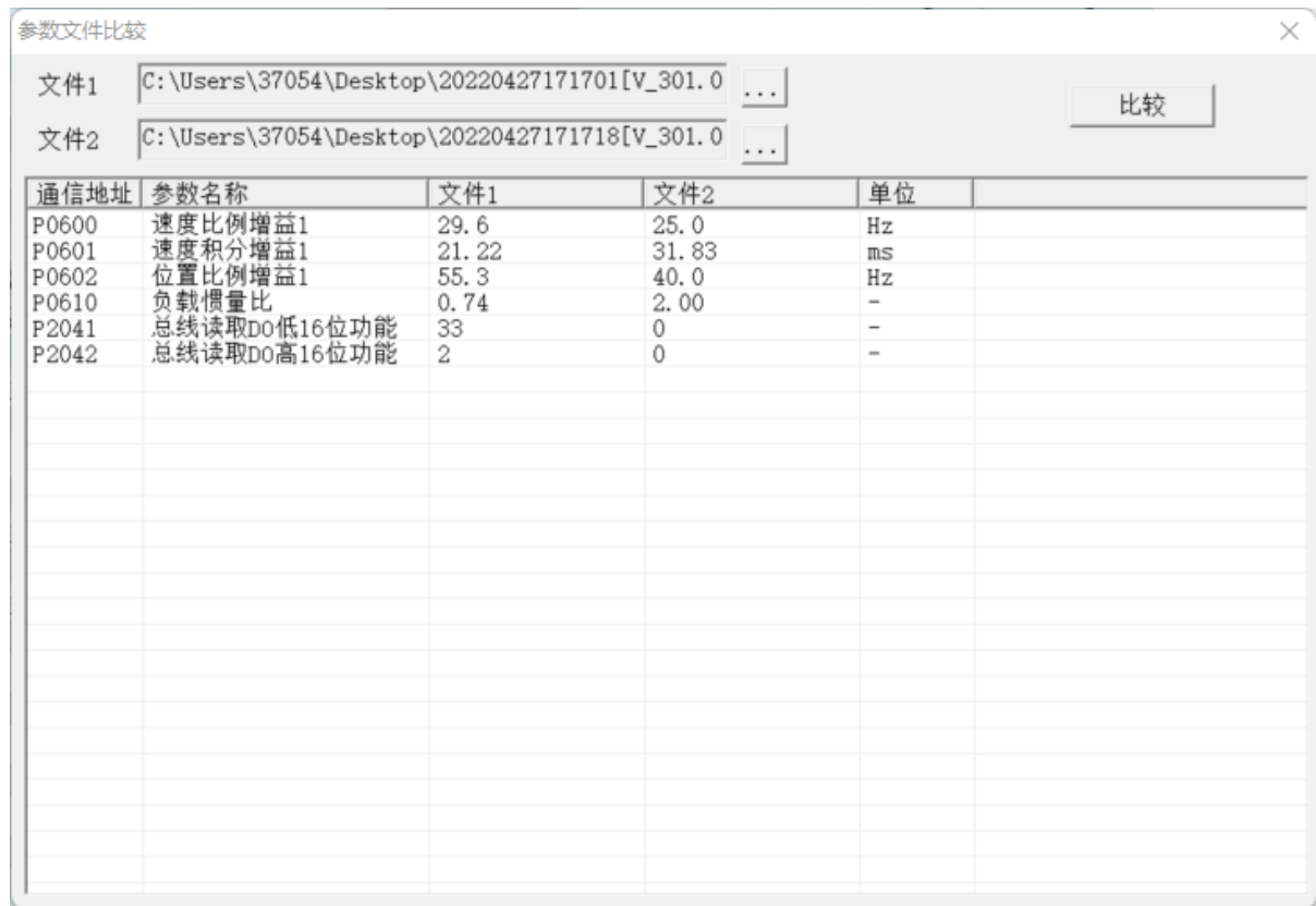
图3-20 参数对比
