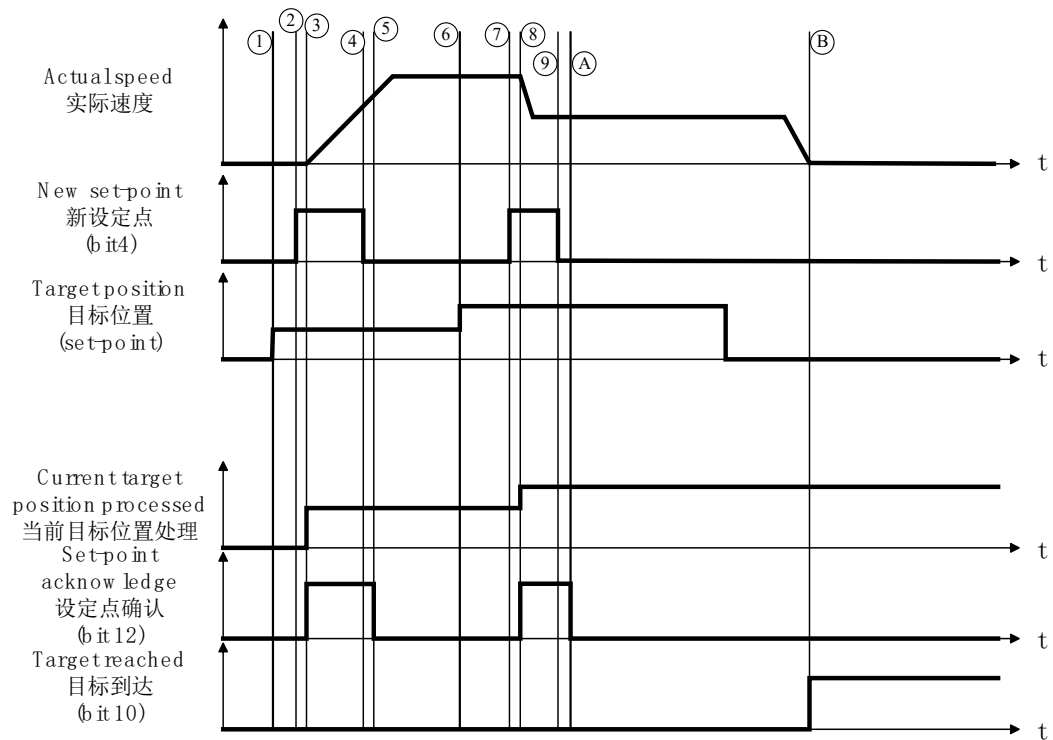
图3-67 PP 模式 Single set-Point (立即更新模式)
