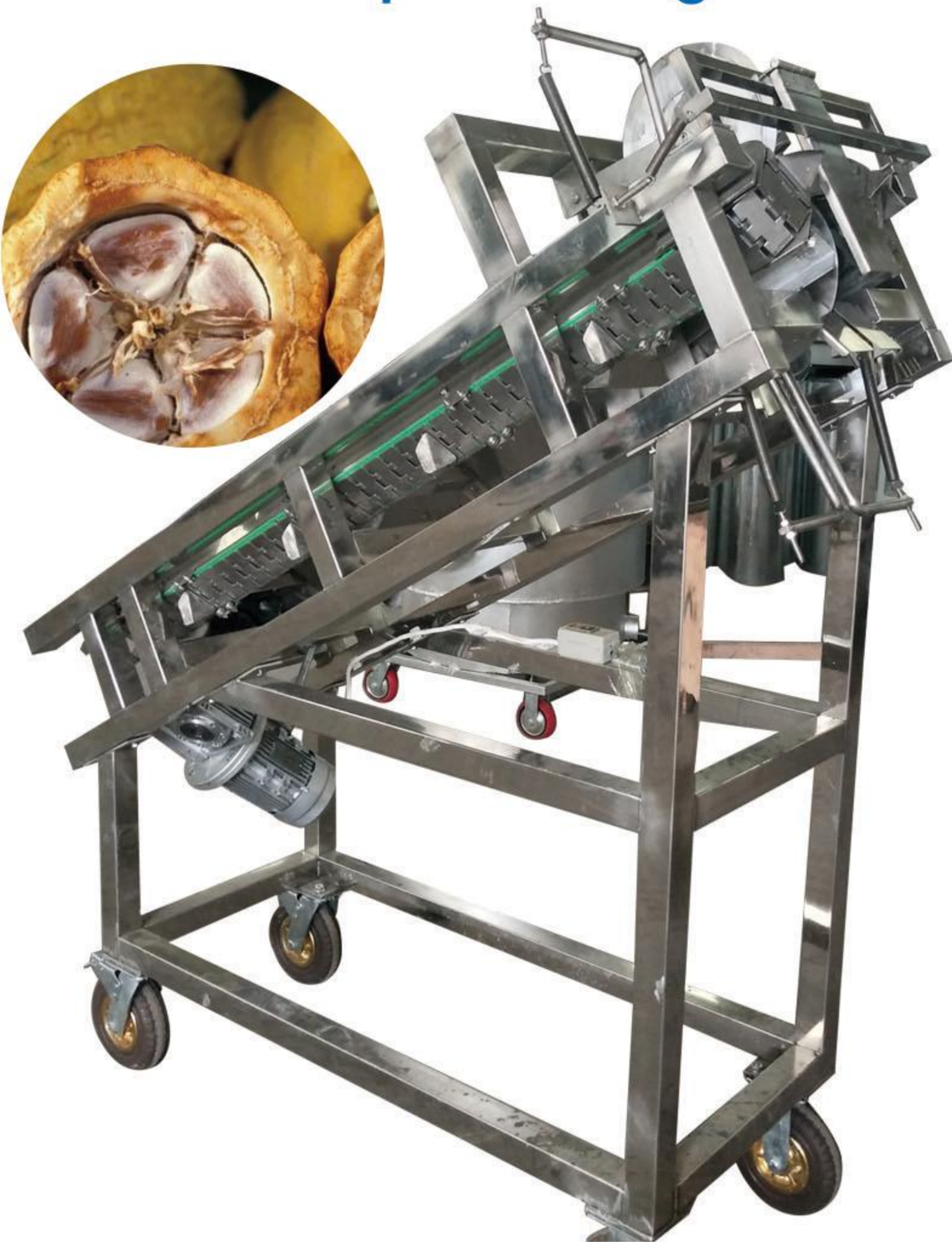
可可荚提升切分机 Cocoa pod lifting cutter
