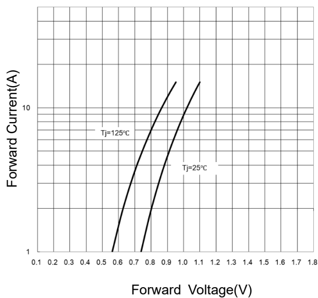
FIG 4: I_F - V_F
