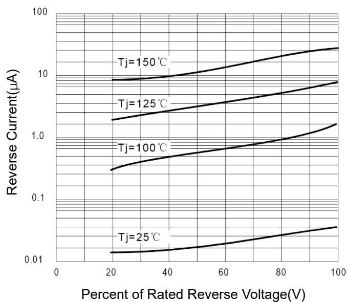
FIG 3: V_R - I_R
