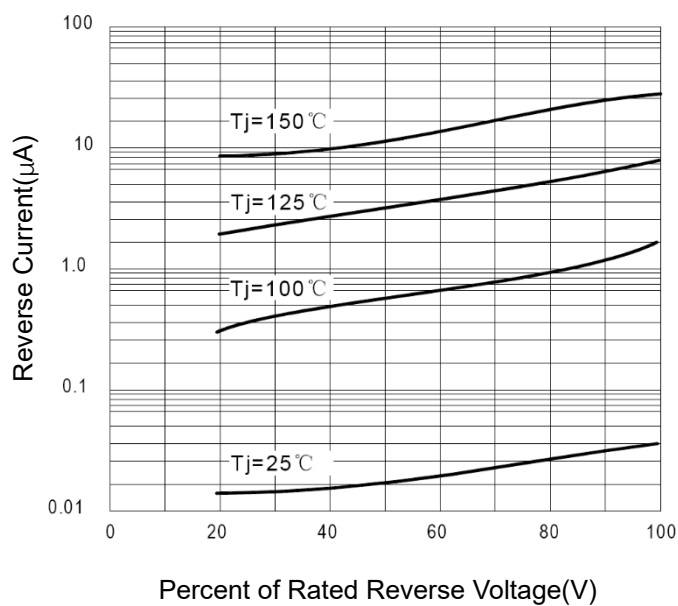
FIG 3: V_R - I_R
