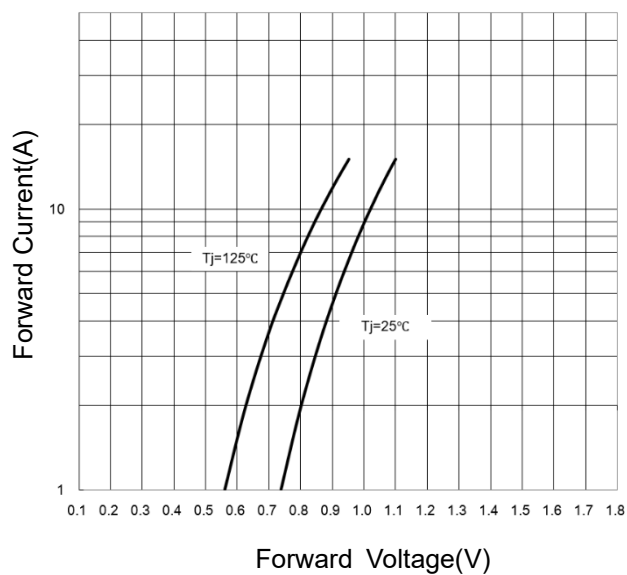
FIG 4: I_F - V_F
