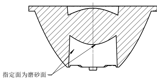
B-B
