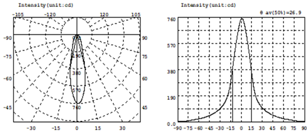
Intensity data: (deg , cd) C0-180
