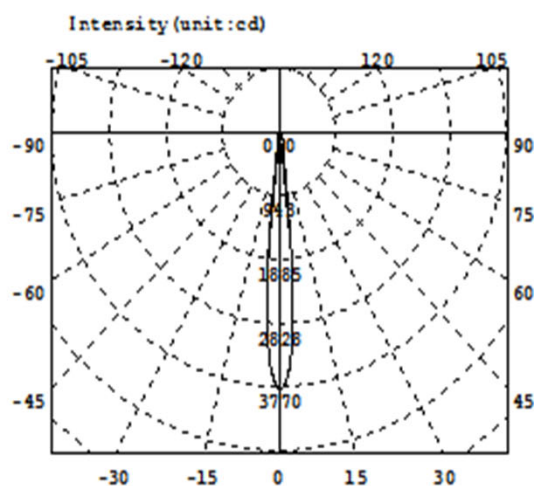
Intensity data: (deg , cd) C0-180
