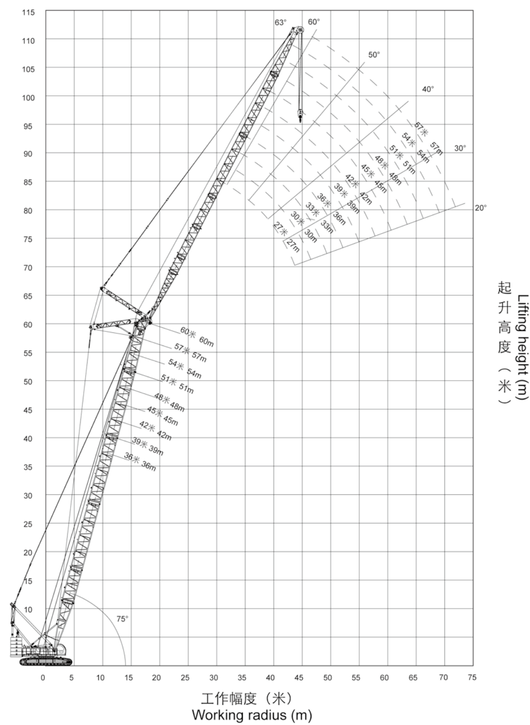
主臂75°时 Boom angle at 75°
