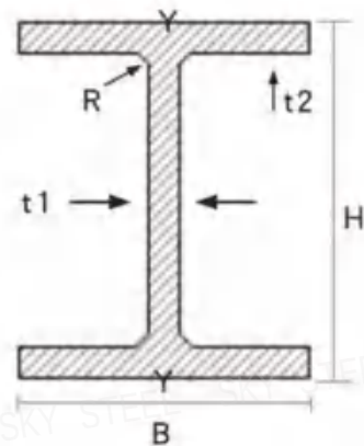
H型钢规格
