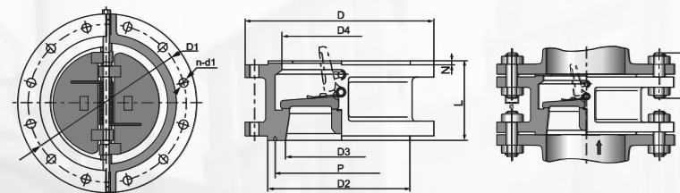
主要连接尺寸 Main Connection Dimension
