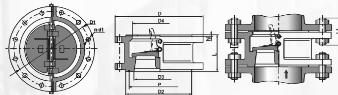
主要连接尺寸 Main Connection Dimension
