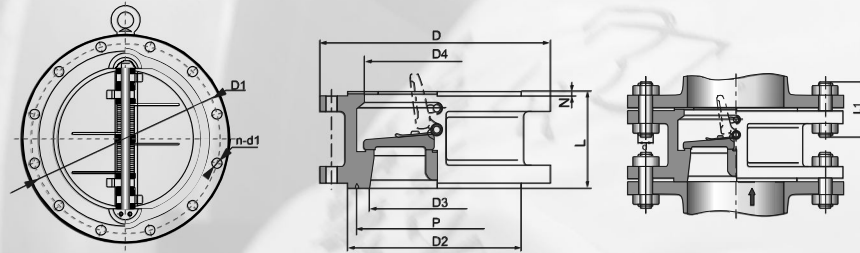
主要连接尺寸 Main Connection Dimension
