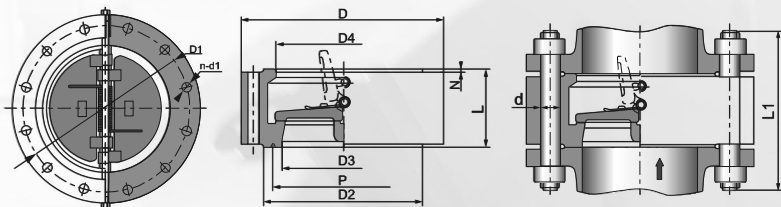
主要连接尺寸 Main Connection Dimension
