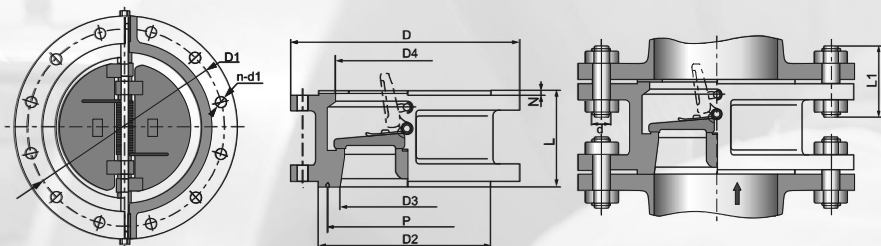
主要连接尺寸 Main Connection Dimension
