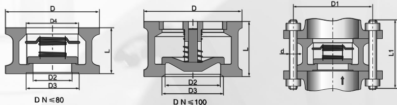
主要连接尺寸 Main Connection Dimension
