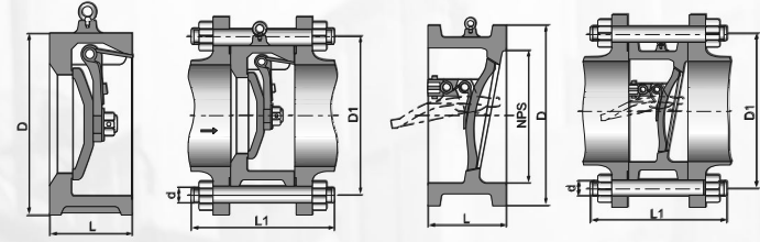
主要连接尺寸 Main Connection Dimension
