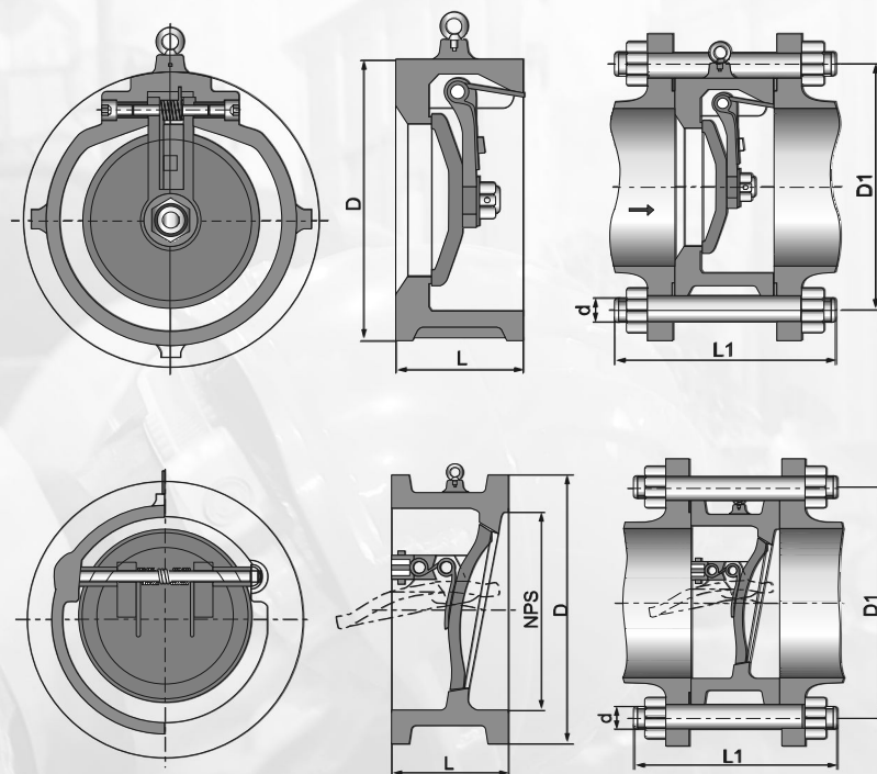
主要连接尺寸 Main Connection Dimension
