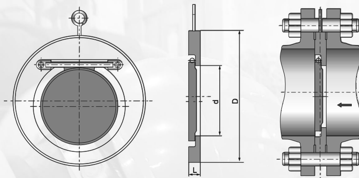
主要连接尺寸 Main Connection Dimension
