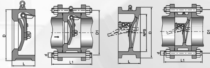
主要连接尺寸 Main Connection Dimension
