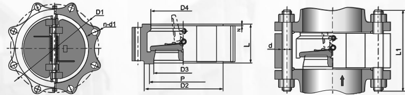
主要连接尺寸 Main Connection Dimension
