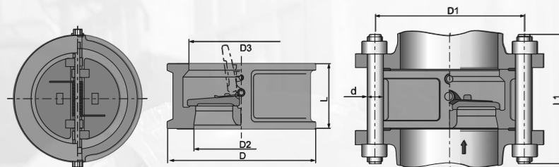
主要连接尺寸 Main Connection Dimension
