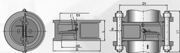
主要连接尺寸 Main Connection Dimension
