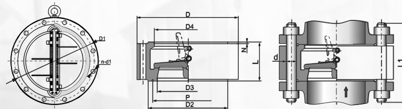
主要连接尺寸 Main Connection Dimension
