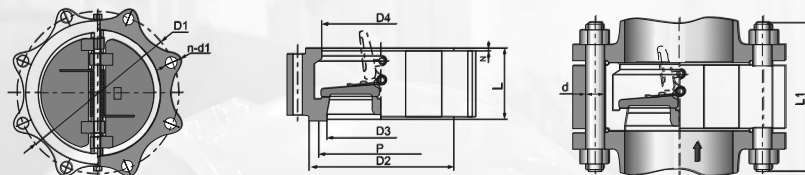
主要连接尺寸 Main Connection Dimension
