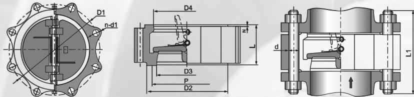
主要连接尺寸 Main Connection Dimension
