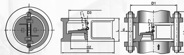
主要连接尺寸 Main Connection Dimension
