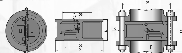
主要连接尺寸 Main Connection Dimension
