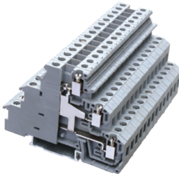
RDIKD 1.5-PV
