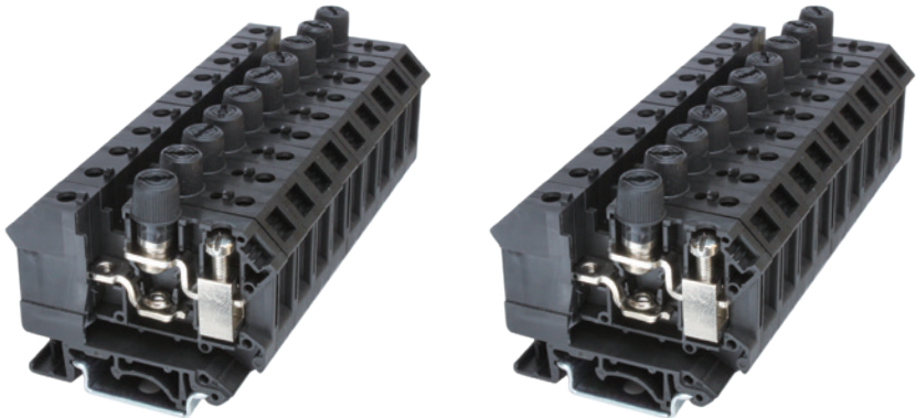
RUK 10 -DREHSI
