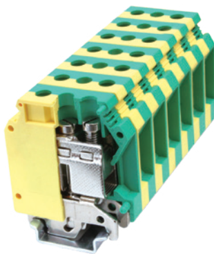
RUSLKG 35N
