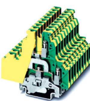
RUKKB 5 -PE
