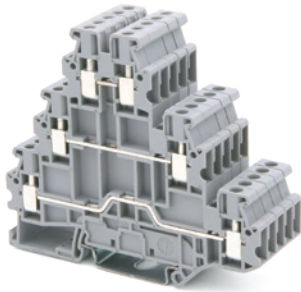
RUT2.5-3L
