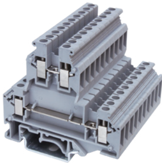
RUKKB 3
