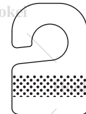
Ref. 352C (500 μ) 2,000 pcs / box 掛鈎厚度: 0.5 毫米 數量: 2,000 個/盒
