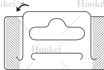
Ref. 410C (380 μ) 2,500 pcs / reel 掛鈎厚度: 0.38 毫米 數量: 2,500 個/卷
