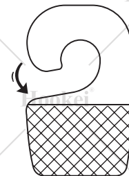
Ref. 361C (500 μ) 3,000 pcs / reel 掛鈎厚度: 0.5 毫米 數量: 3,000 個/卷
