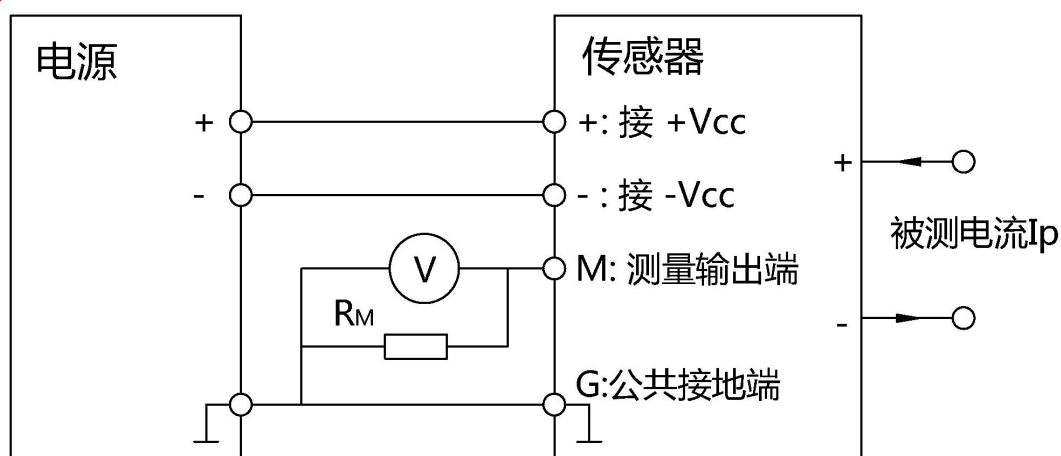
电连接示意图
