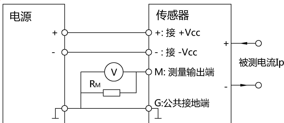
电连接示意图
