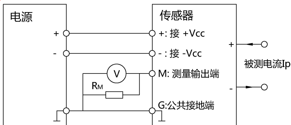
电气连接示意图
