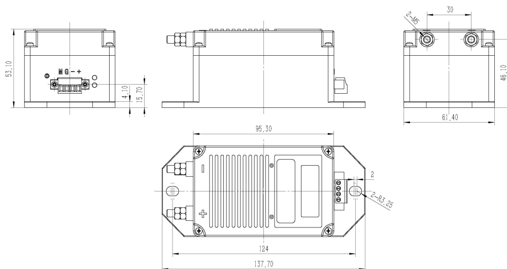
Чертеж внешних размеров
