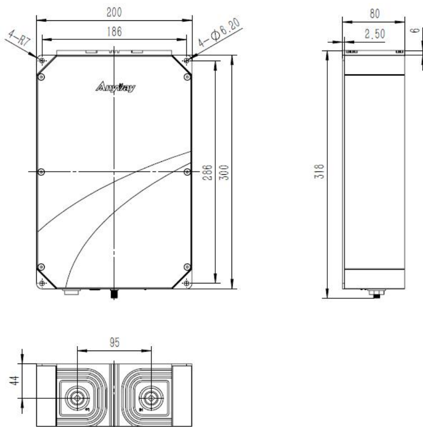
Чертеж внешних размеров
