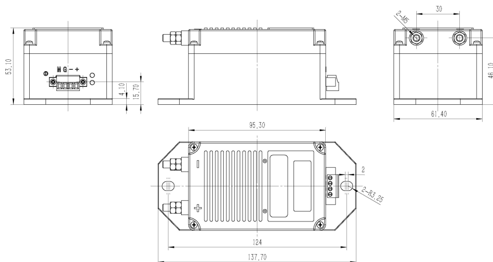
图 1 外观尺寸图
