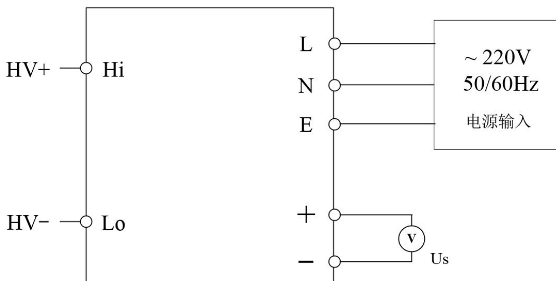
图 3 电气连接图
