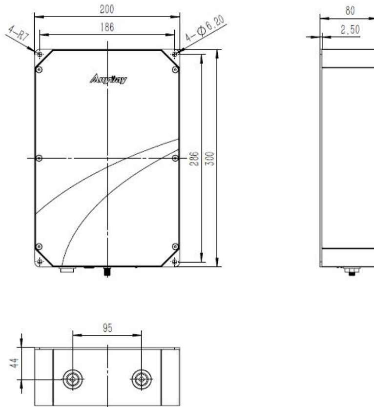
Чертеж внешних размеров
