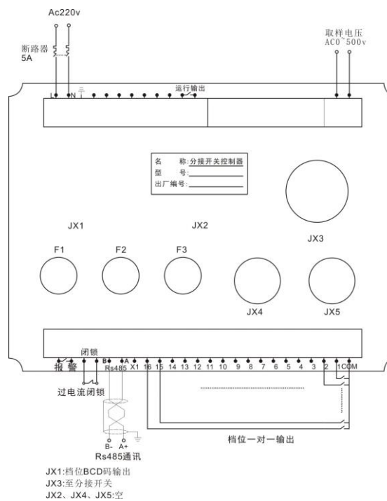
后面板接线图
