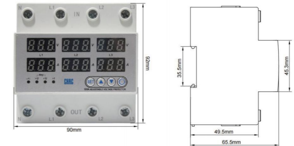
3P+N 100A
