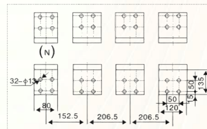
Vertical Busbar (垂直接线)
