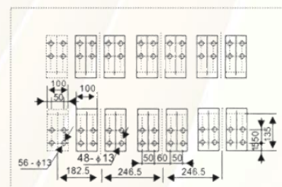
Vertical Busbar (垂直接线)
