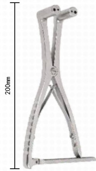
Q7-14 克氏针撑开器 II Kirschner Forceps Distractor II 孔直径: \Phi 1.6 + \Phi 2.5
