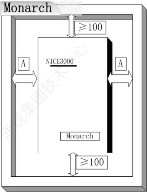
图4-2 控制器的安装尺寸要求
