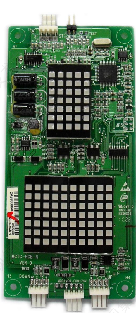
图3-3-13 MCTC-HCB-N实物图
