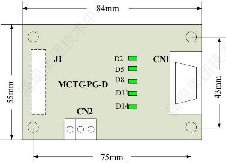
图4-8 MCTC-PG-D外观及尺寸
