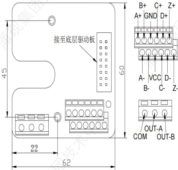
图4-9 MCTC-PG-C（ERN1387型编码器）
