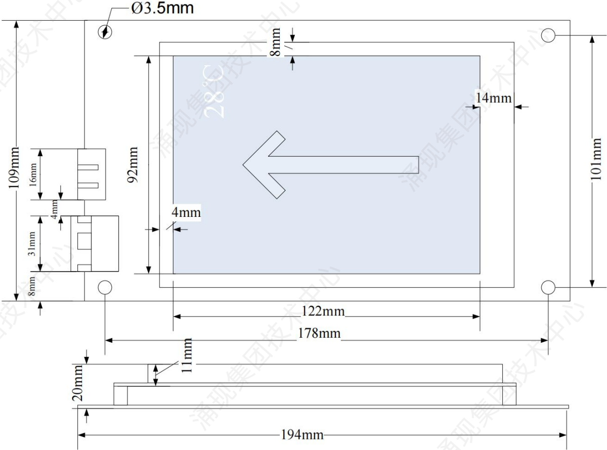
图3-3-16 MCTC-HCB-K安装尺寸
