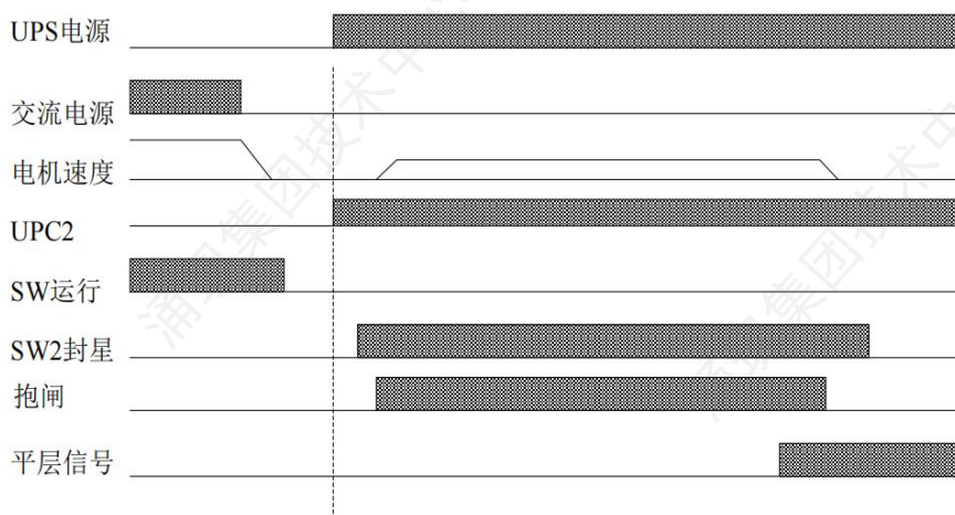
图7-5 自溜车时序
