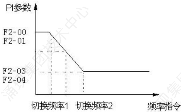
图6-3 PI参数示意图
