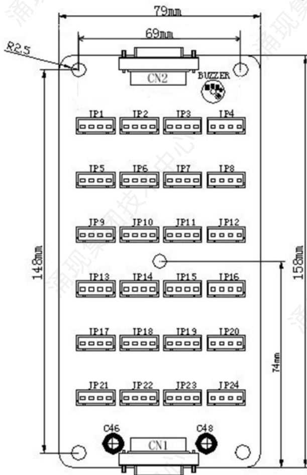
图3-2-1 指令板安装尺寸
