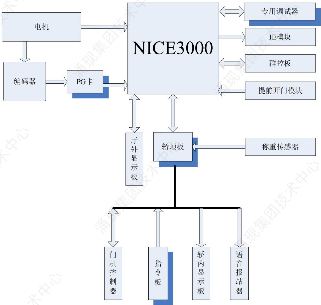
图3-1 NICE3000控制系统图
