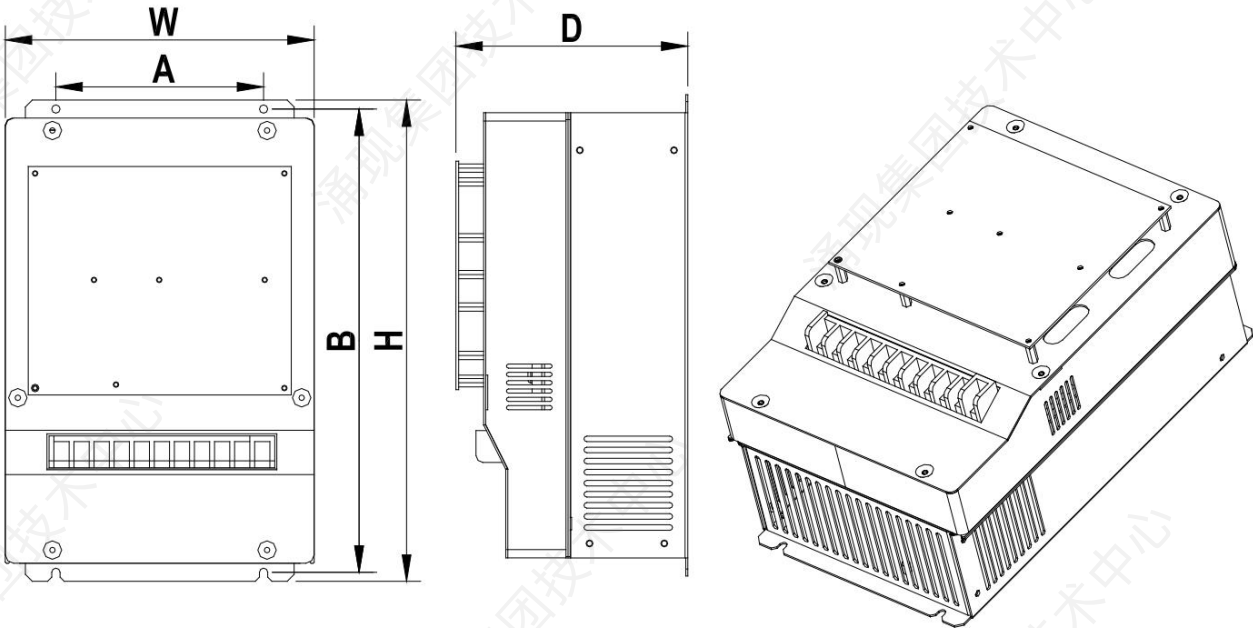
图2-4-1 控制器外观及尺寸示意图
