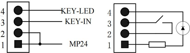
图3-2-3 4PIN接口定义及外部接法
