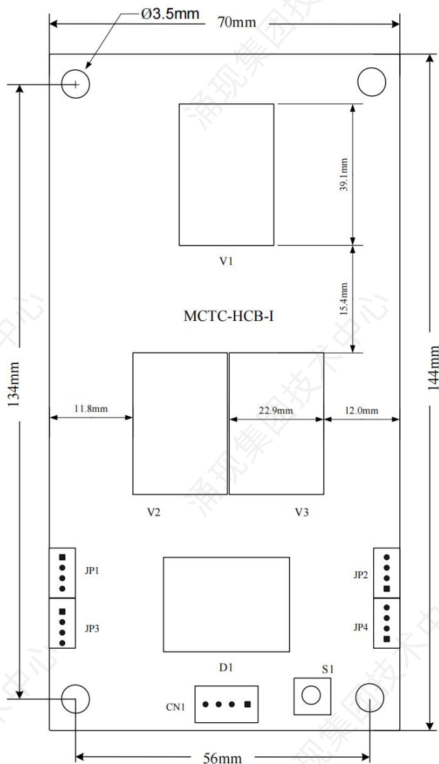
图 3-3-12 MCTC-HCB-I 安装尺寸
