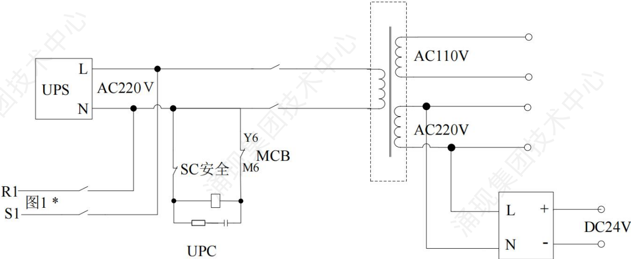
2) UPS电源回路图
