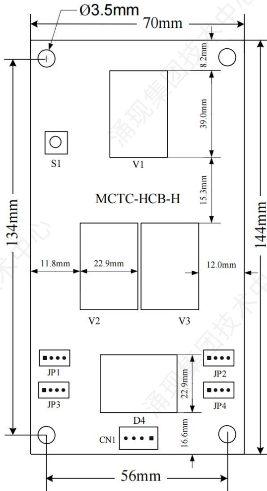
图3-3-10 安装尺寸
