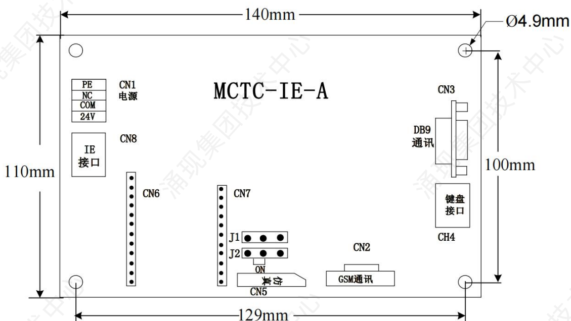
图3-8-1 MCTC-IE-A安装尺寸图
