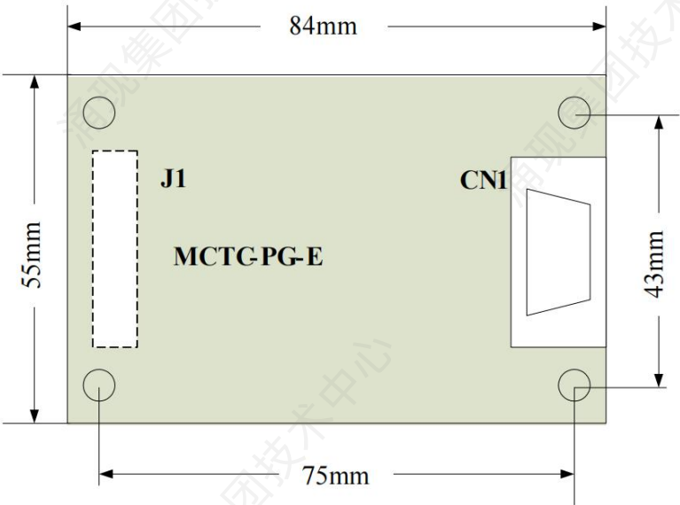
图4-11 MCTC-PG-E外观及尺寸
