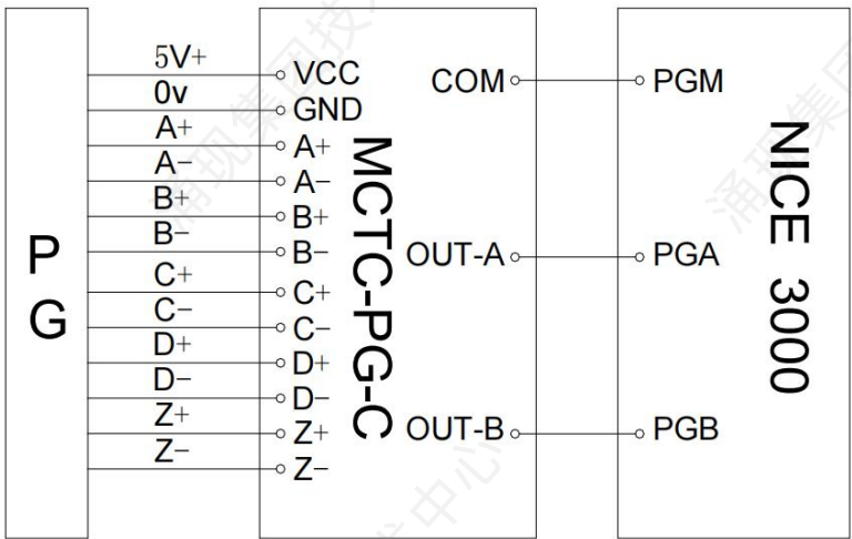
图4-10 MCTC-PG-C接线图（ERN1387型编码器）
