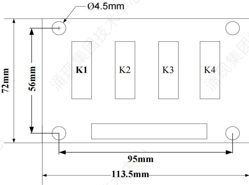
图3-5-2外观尺寸图
