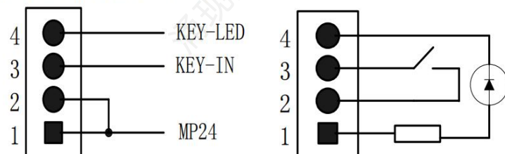
普通按钮输入端子 (JP1-4)
