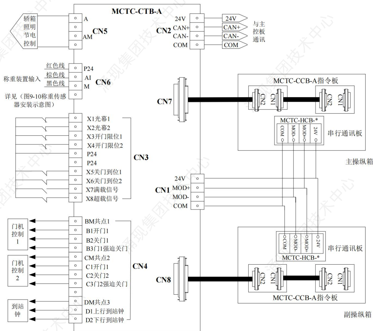
图7-3 轿顶板推荐接线
