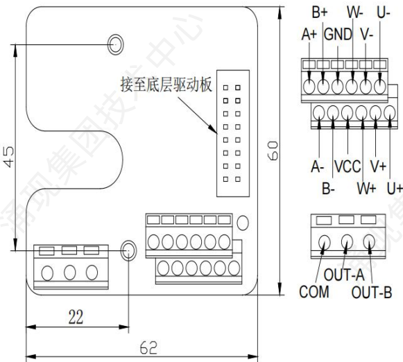
图4-6 MCTC-PG-B示意图
