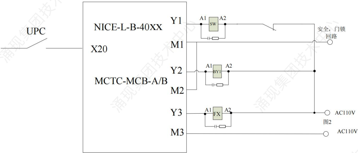
图7-4 停电应急运行系统示意图
