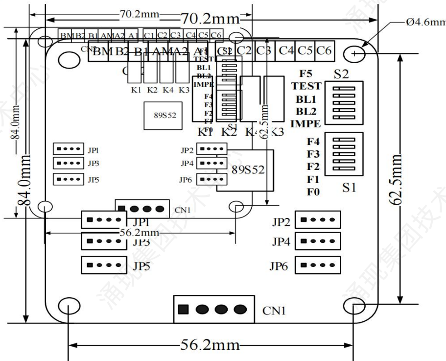
图3-3-2 MCTC-HCB-B安装尺寸图
