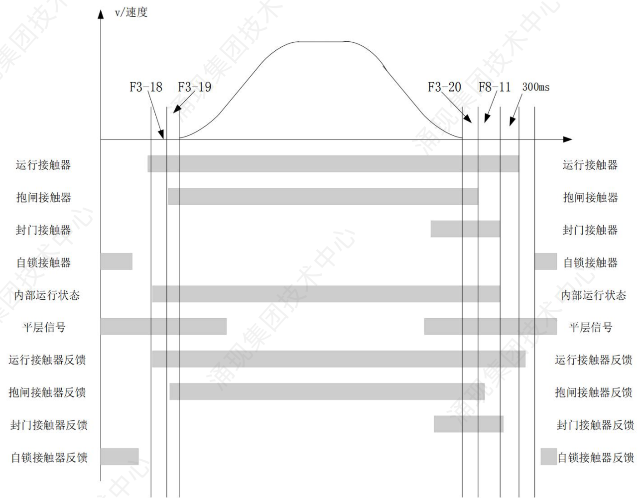
图6-5 运行时序图
