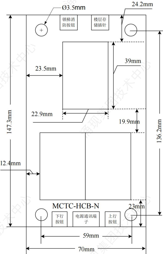
图3-3-14 MCTC-HCB-N安装尺寸
