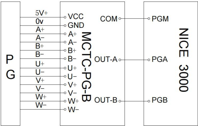
图4-7 MCTC-PG-B接线图
