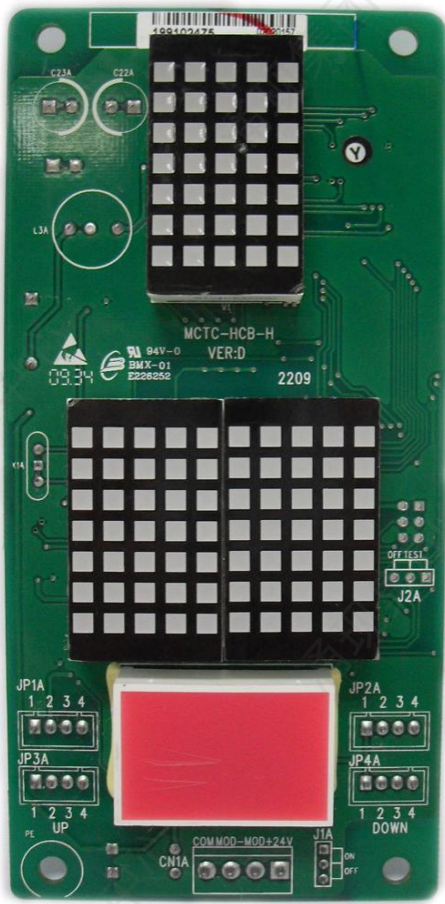
图3-3-9 MCTC-HCB-H实物图
