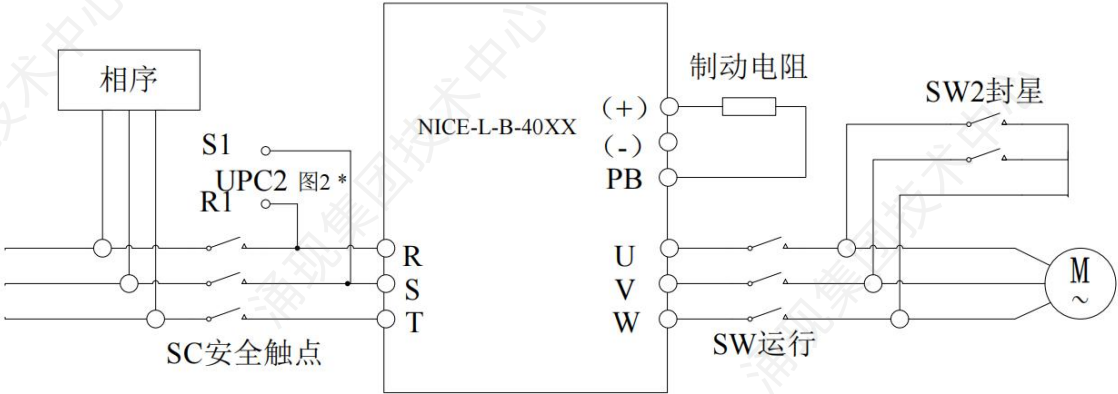
2) UPS电源回路图
