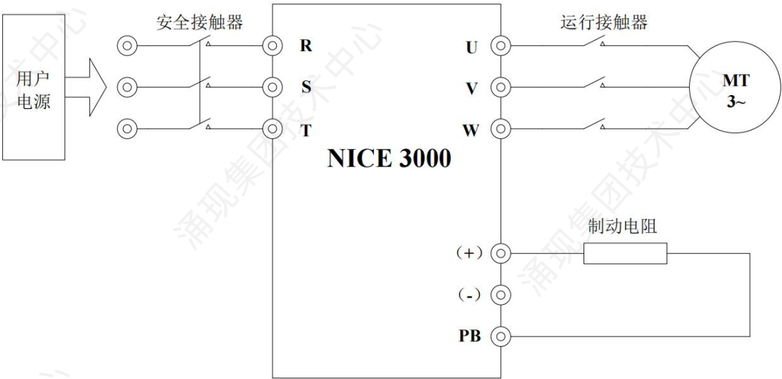
图4-3 主回路接线图
