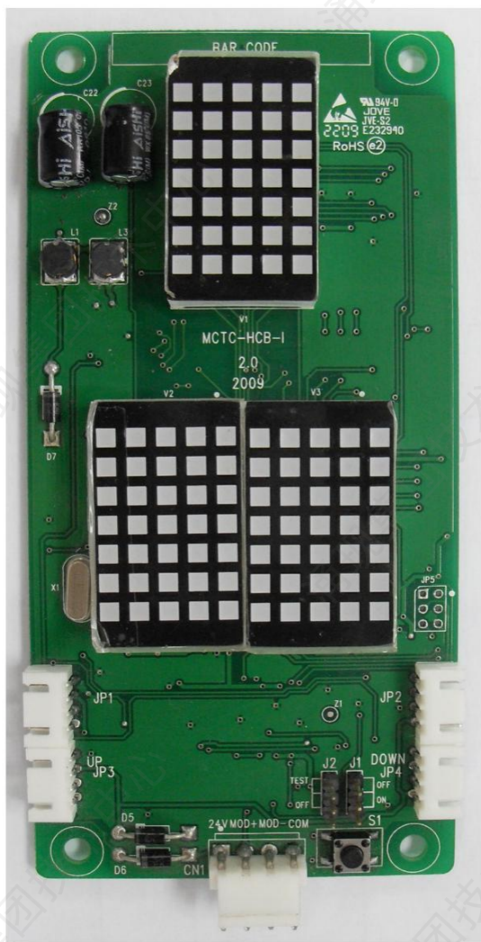
图 3-3-11 MCTC-HCB-I实物图
