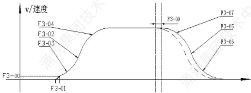
图6-4 速度曲线图
