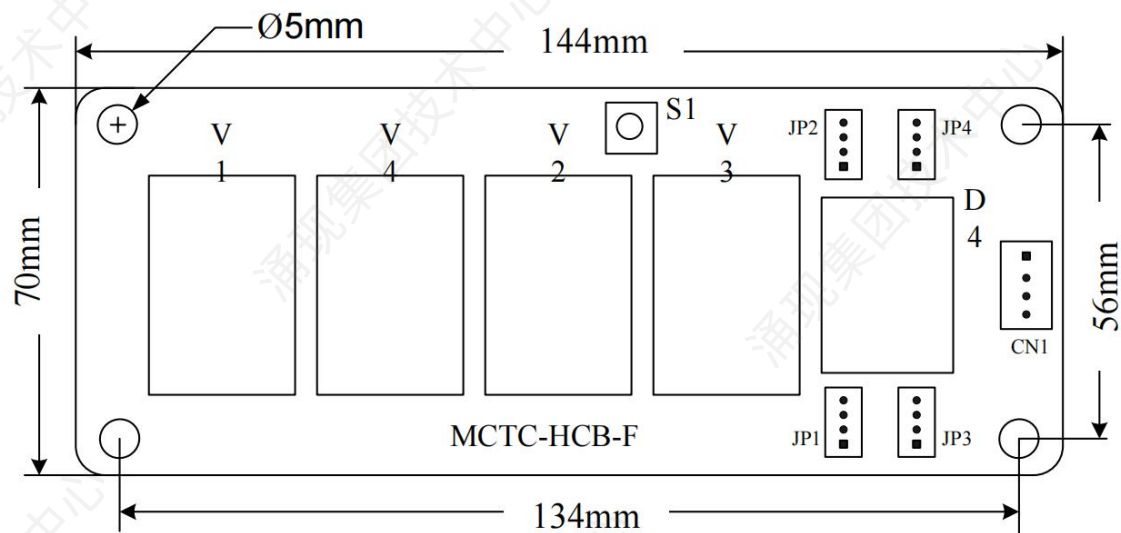
图3-3-8 MCTC-HCB-F安装尺寸
