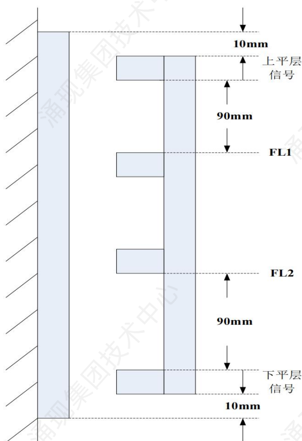
图3-5-3上下再平层门区感应器安装方法
