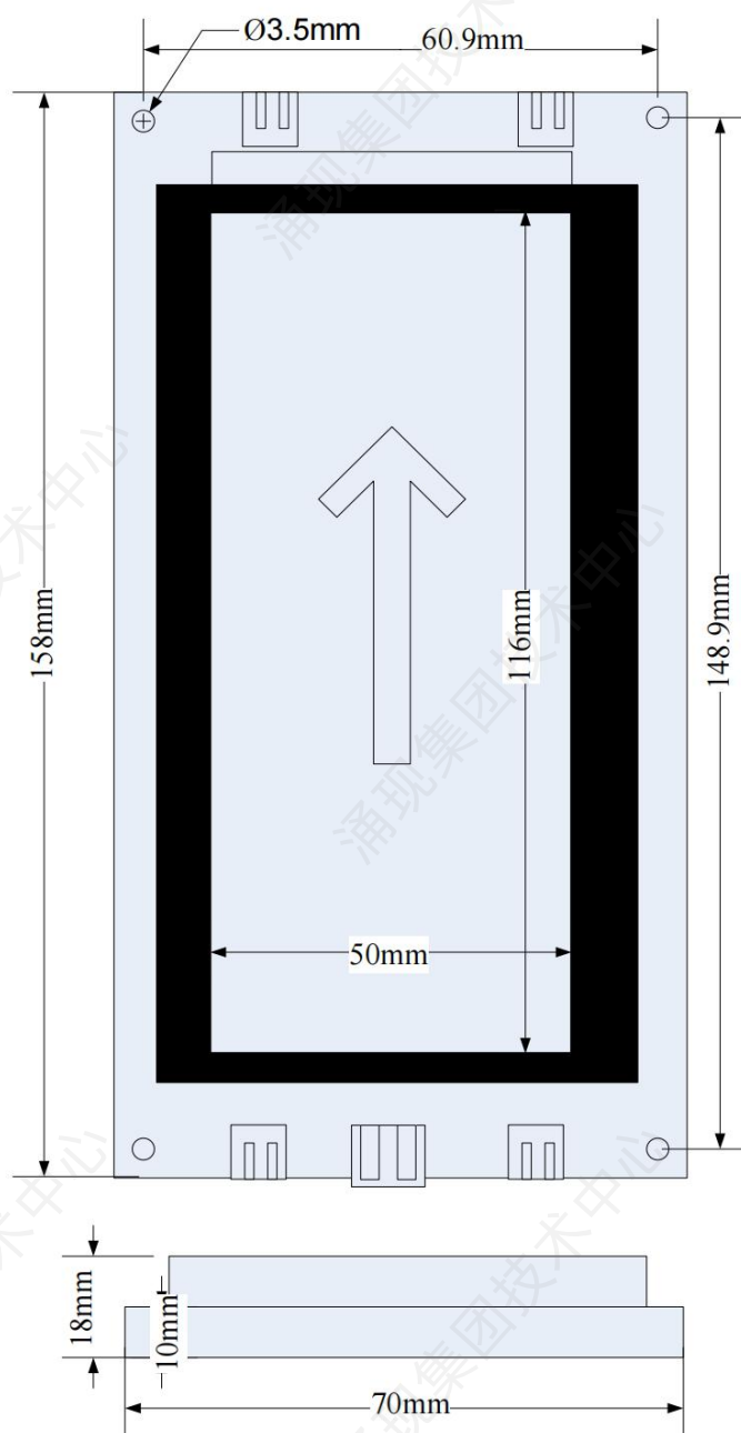
图3-3-6 MCTC-HCB-D1尺寸图
