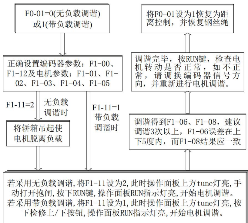
图6-2 同步电机调谐流程图
