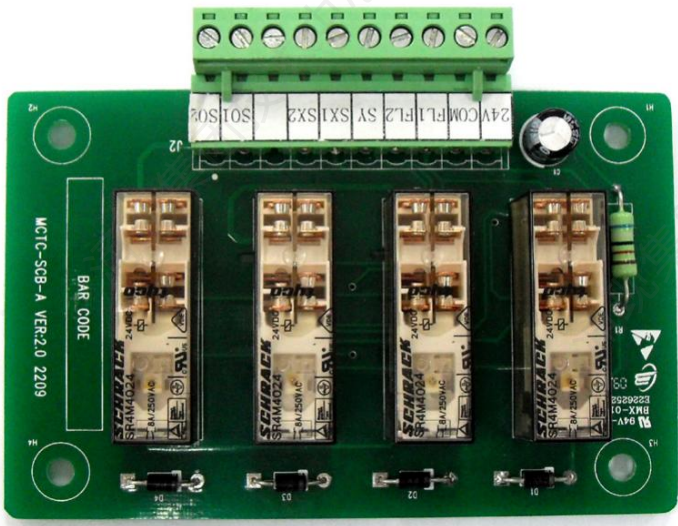
图3-5-1 实物图
