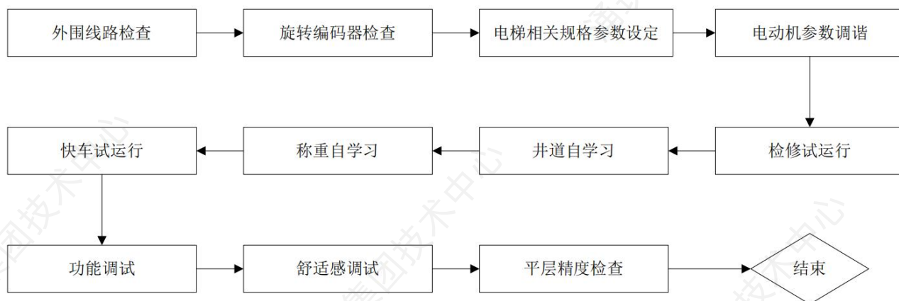
图7-1 调试流程
