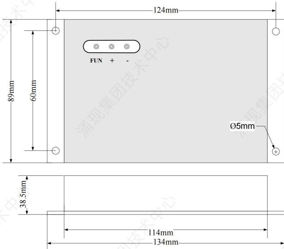
图 3-6-1 MCTC-CHM-B 尺寸图
