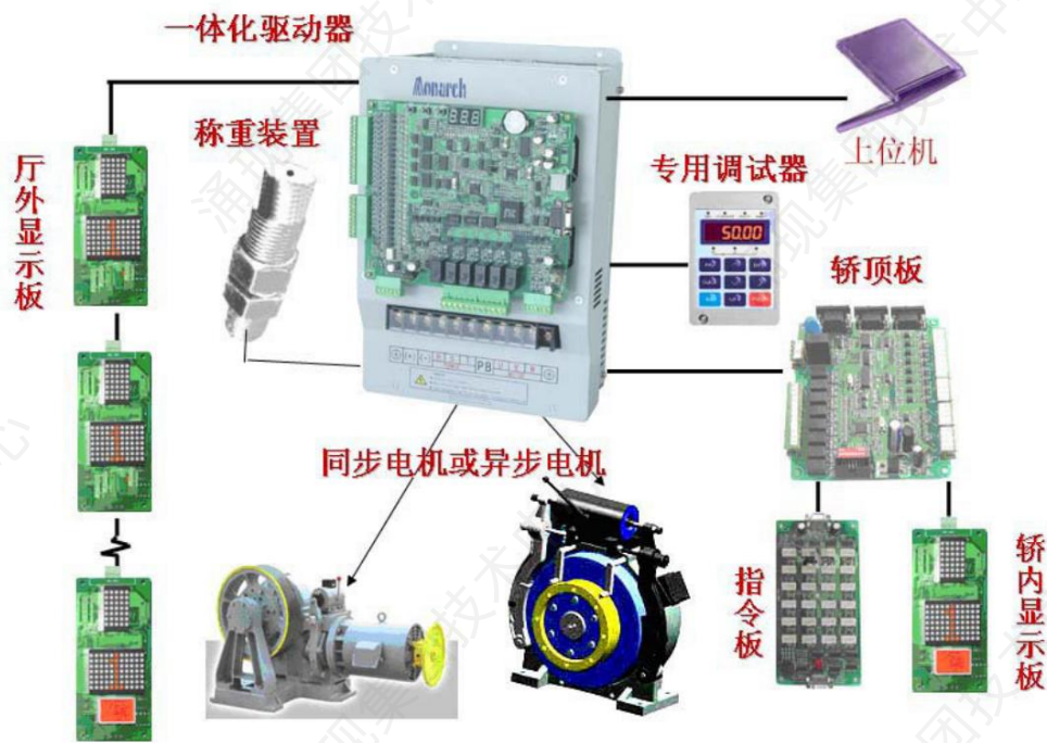
图 4-1 系统配置简图
