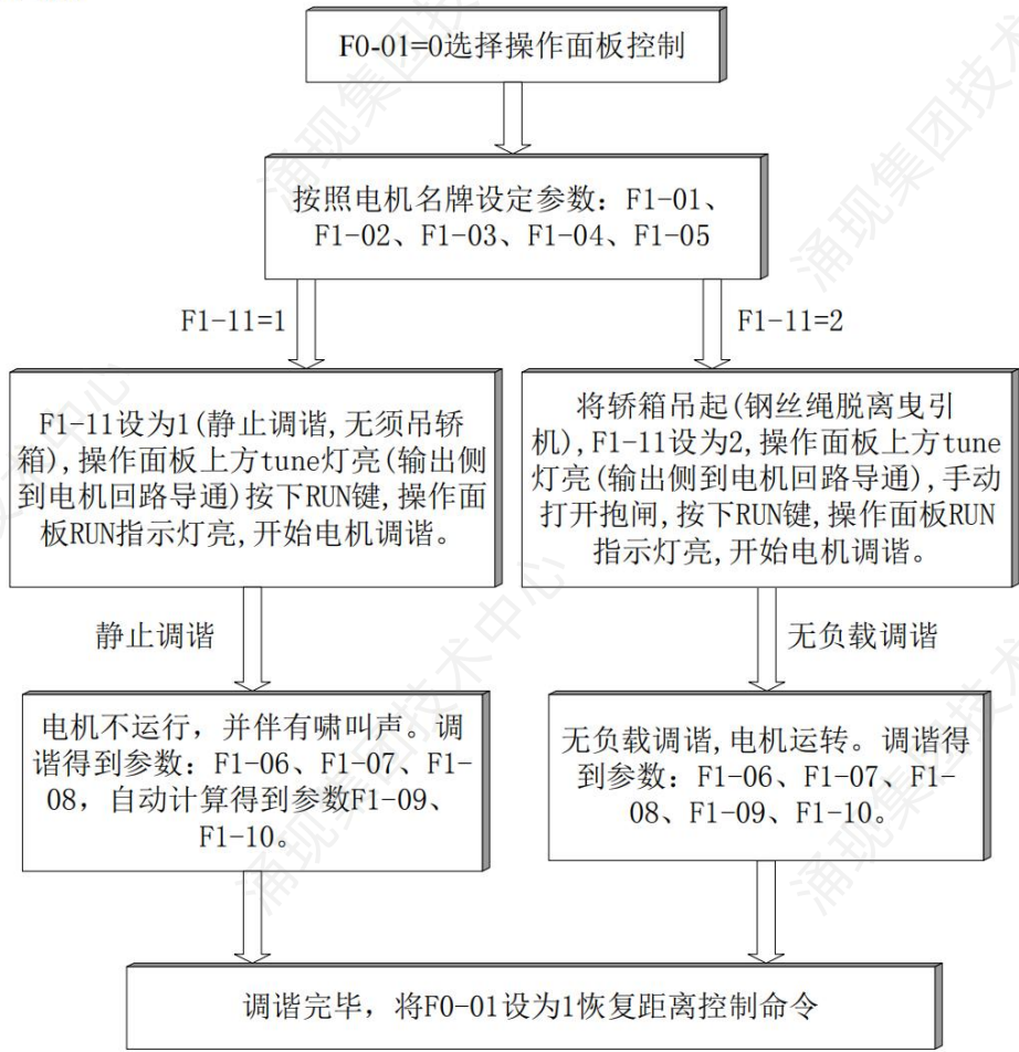
图6-1 异步电机调谐流程图
