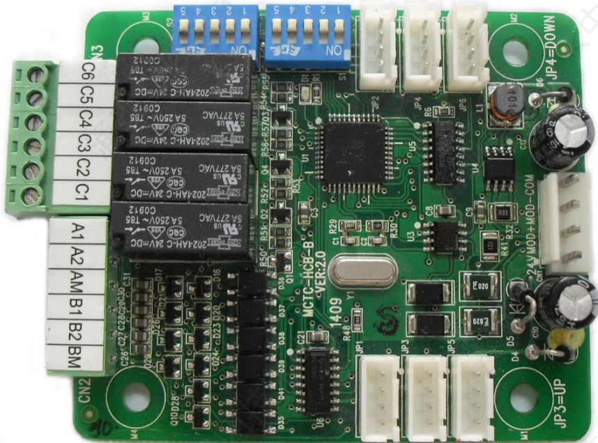
图 3-3-1 MCTC-HCB-B实物图
