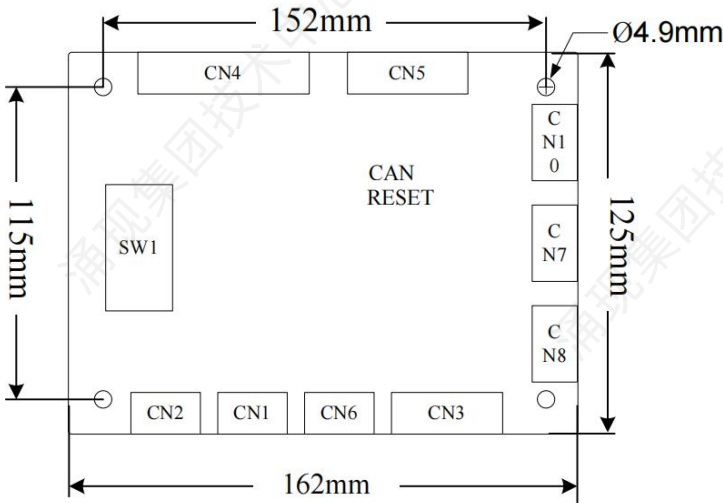
图3-1-1 轿顶板安装尺寸
