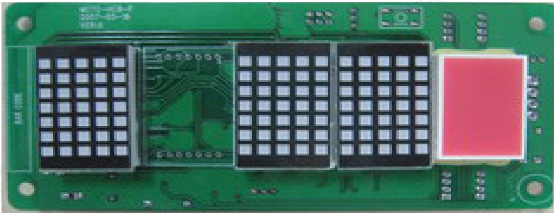
图 3-3-7 MCTC-HCB-F实物图
