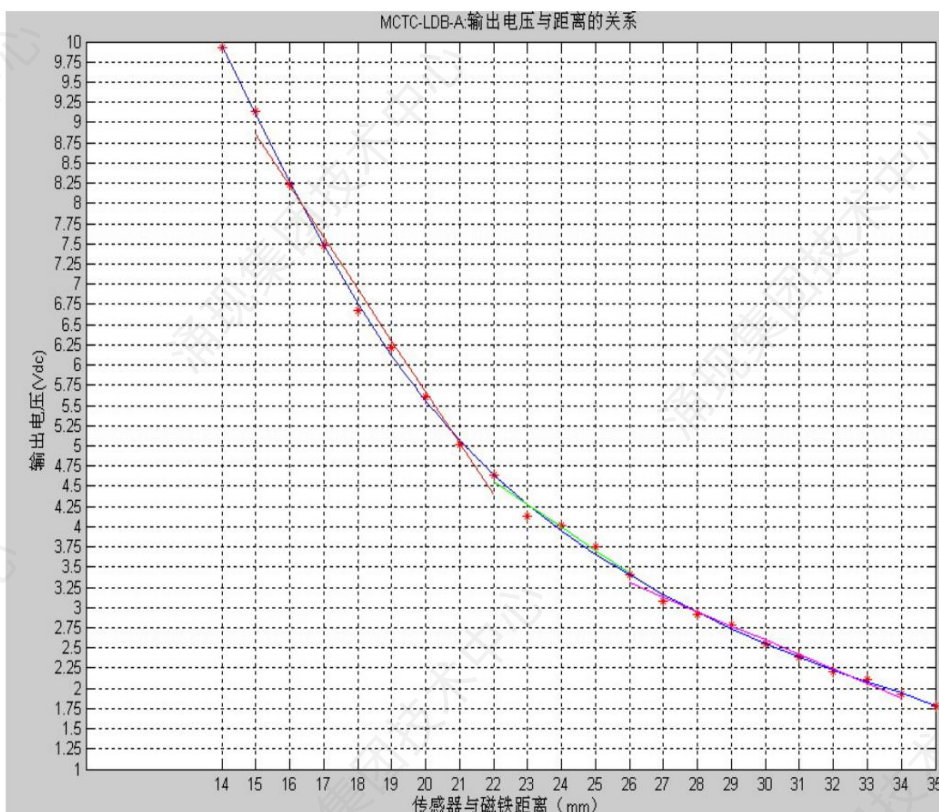
图3-7-3称重传感器输出电压示意图
