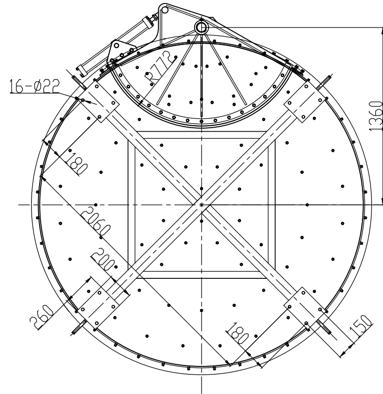
底脚安装尺寸图
