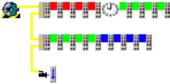
Fig. 248: Simple I/O topology
