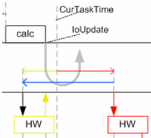
Fig. 271: Local slave shift time
