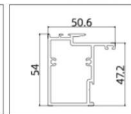
GH-TM21045(Striker Stile)
