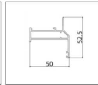
LB-PK5003-1.35 (Sash)
