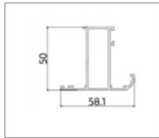
BG-PC50103 (Sash)
