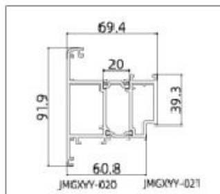
JMGXYY-GPM65103 (Sash)
