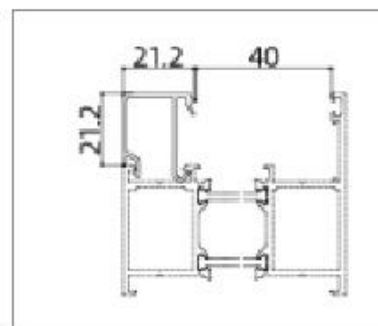
APG70F040 (Sash)
