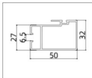
AB8012-1.35A (Striker Stile)
