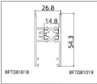
Door Rail
