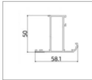
BG-PC50103 (Sash)
