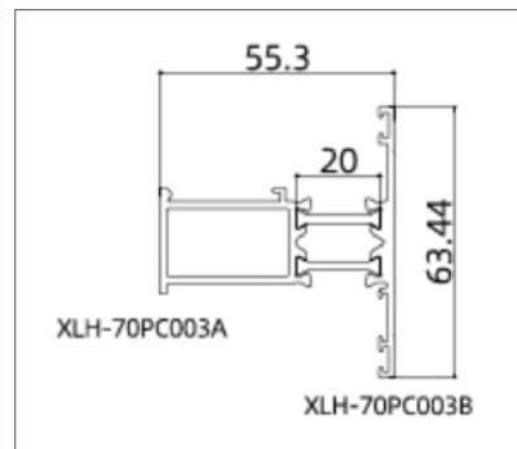
XLH-70PC003 (Sash)
