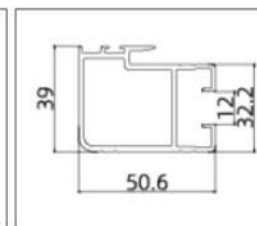
GH-TM21035 (Striker Stile)
