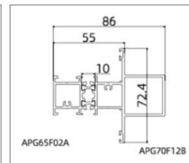
APG60F012(Mullion)
