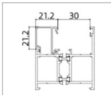
SHZX-PC501023 (Sash)
