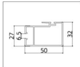
AB8012-1.35 (Striker Stile)
