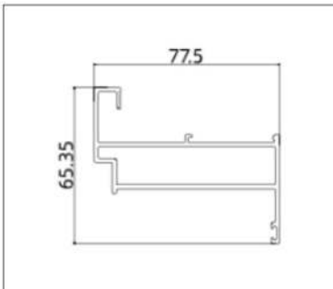
ALP7003 (Sash)
