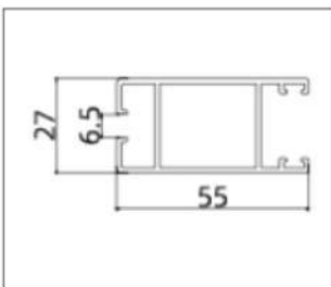
AB8013-1.35 (Striker Stile)
