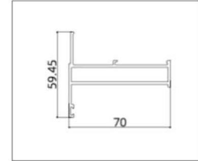
ALP7003(Sash)
