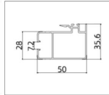
AK8207 (Striker Stile)
