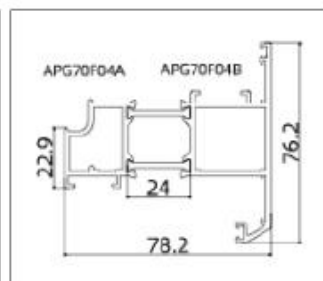
APG70F04 (Sash)
