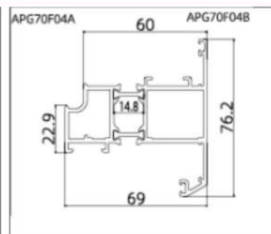
APG60F04 (Sash)
