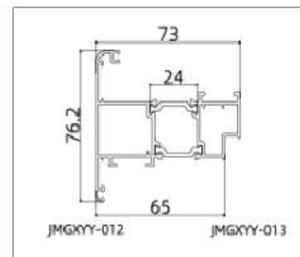
JMGXYY-GPC65103 (Sash )
