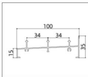
AB8016 ( Track)
