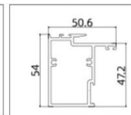
GH-TM21045 (Striker Stile)
