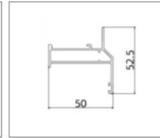
LB-PK5003-1.35 (Sash)
