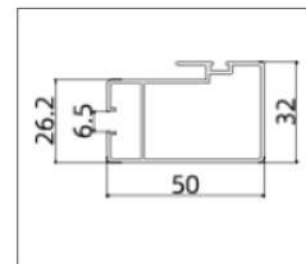
AB8012-0.95( Striker Stile)
