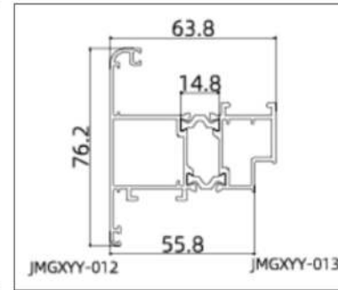
JMGXYY-GPC55103 (Sash)
