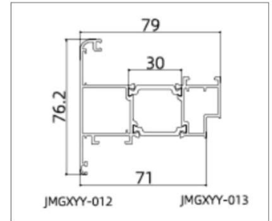
JMGXYY-GPC70103 (Sash)
