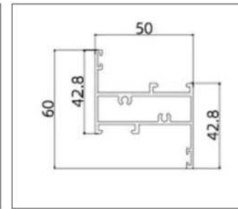
AL-PKC5002A (Z Mullion)
