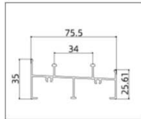
AB805-1.2 ( Track)
