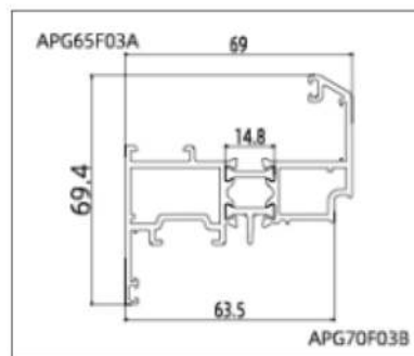
APG60F03 (Sash)
