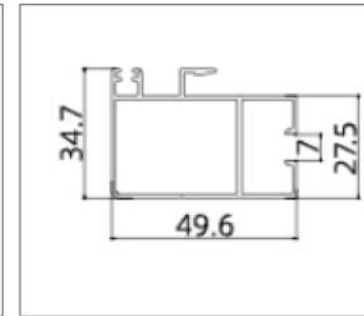
GH-85T06(Striker Stile)
