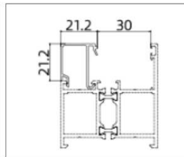
APG70F040 (Sash)
