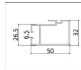
AB8012-1.15 (Striker Stile)
