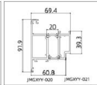
JMGXXY-GPM60103 (Sash)
