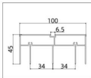
AB8015 ( Track)
