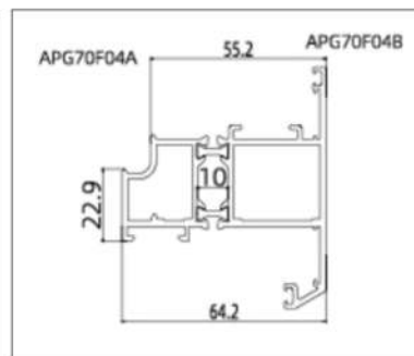
APG55F04 (Sash)
