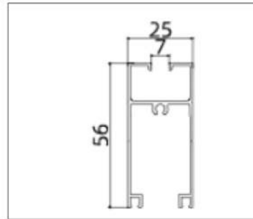
GH-85T04 (Door Rail)
