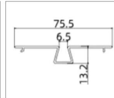
AB8009( Interlock)
