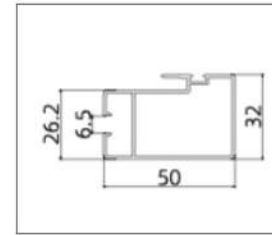
AB8012-0.95 (Striker Stile)
