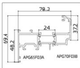
APG70F03 (Sash)
