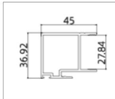
XLH-85TC011 ( Striker Stile)
