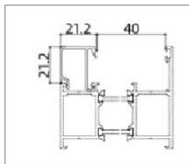
APG70F040 (Sash)
