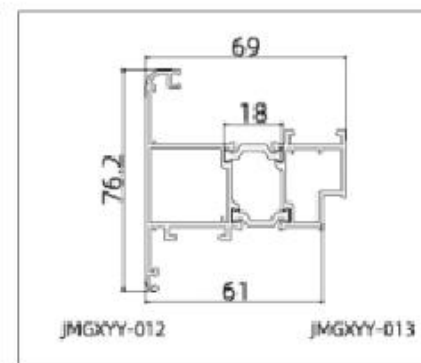
JMGXYY-GPC60103 (Sash)
