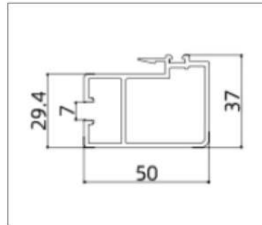
A8211-1.8 (Striker Stile)
