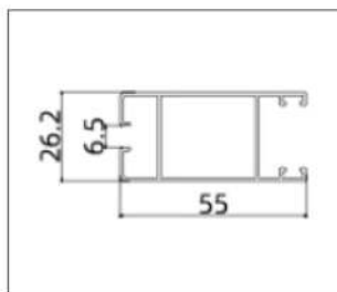
AB8013-0.95 (Striker Stile)
