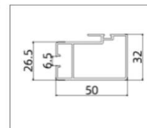
AB8012-1.15( Striker Stile)
