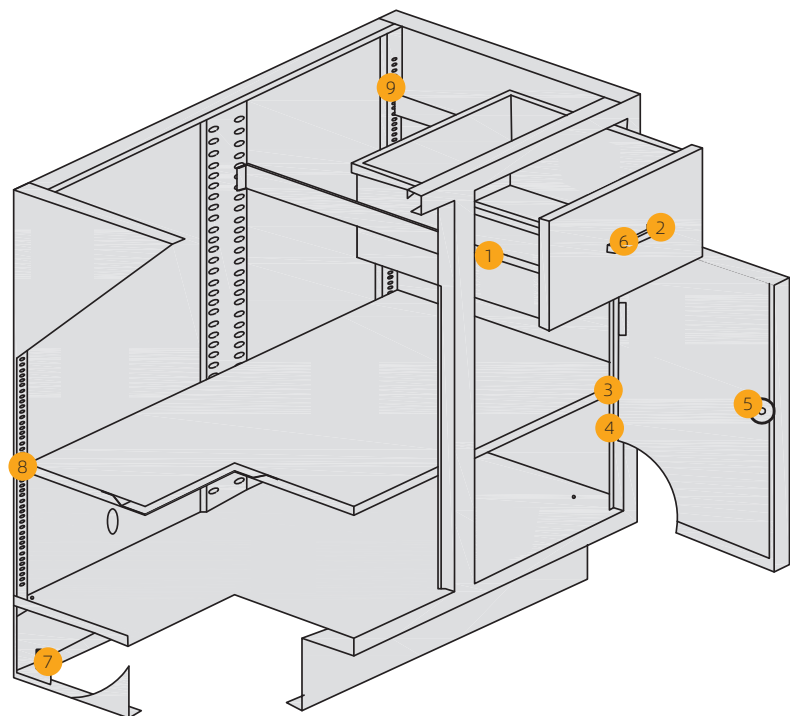
6 PP拉手 GLSP-1209 Plastic Handle
