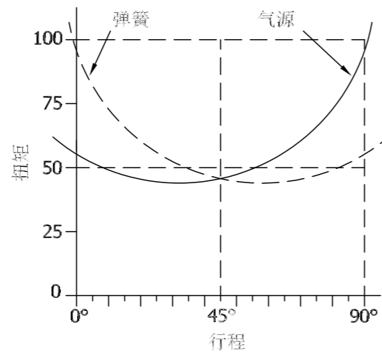
单作用扭矩曲线
