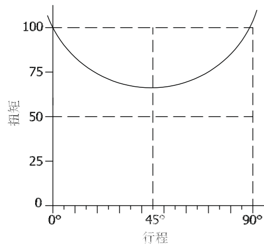
双作用扭矩曲线
