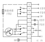
图1 110/220VAC普通开关型
