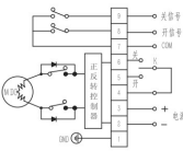
图5 直流正反控制型
