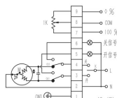
图2 110/220VAC带电位器输出型
