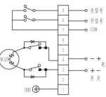
图4 直流普通开关型
