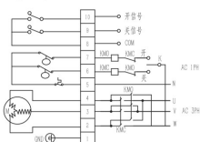
图8 380VAC普通开关型
