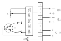
图3 110/220VAC基本调节型
