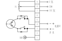
图6 直流带电位器输出型
