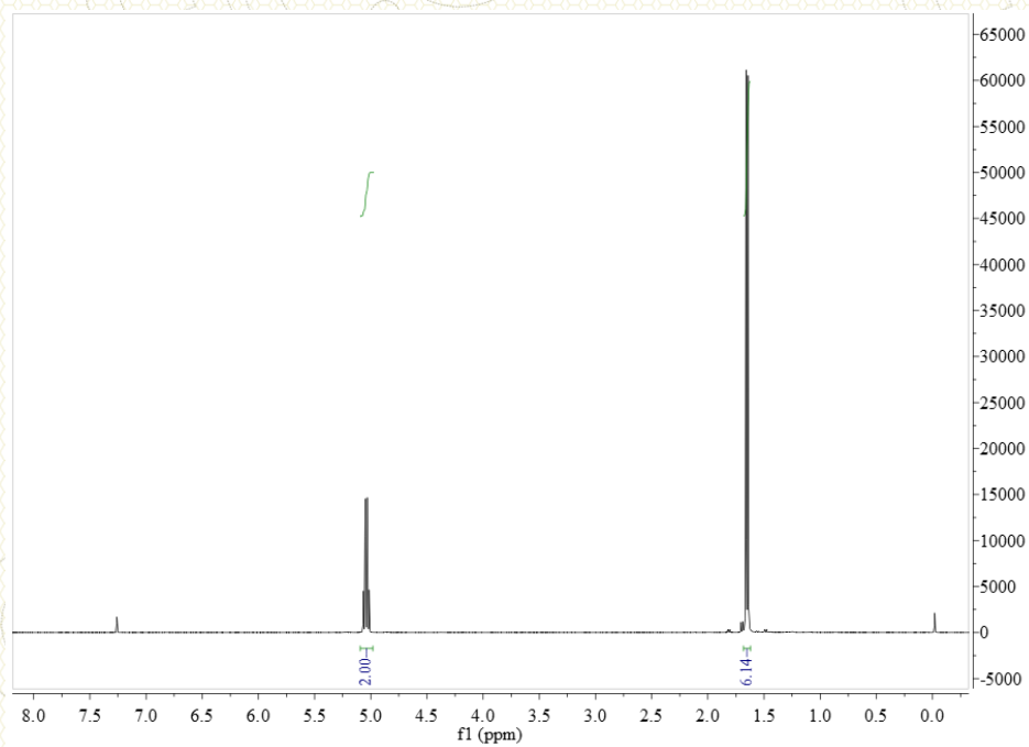
图 1-1 原样的 NMR 测试图
