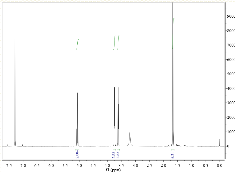
图 1-2 原样内标的 NMR 测试图
